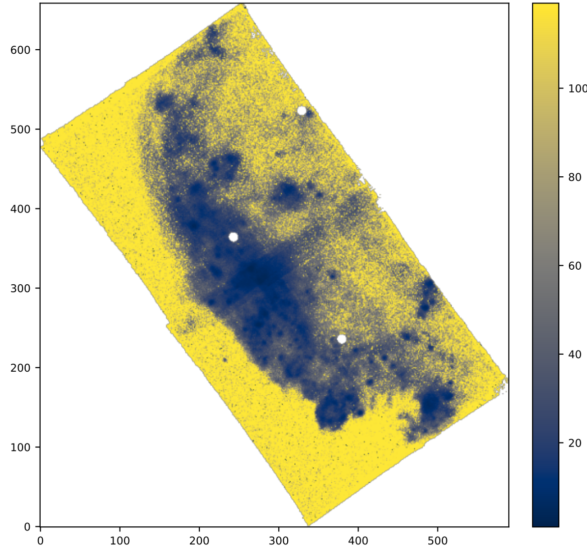
SPAXELS NII6583_SIGMA_ERR
