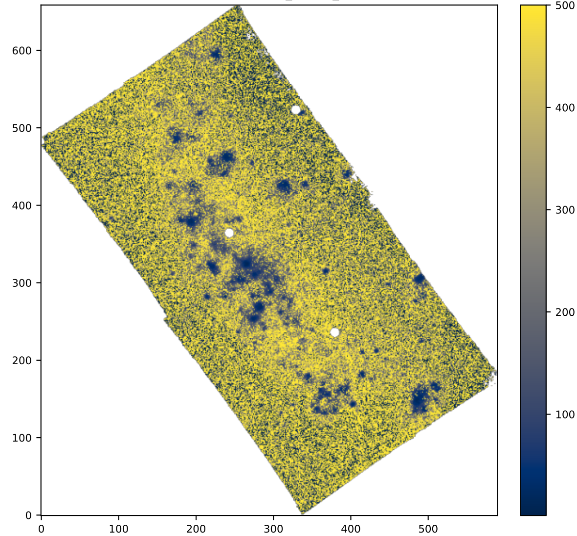
SPAXELS OIII5006_SIGMA_ERR
