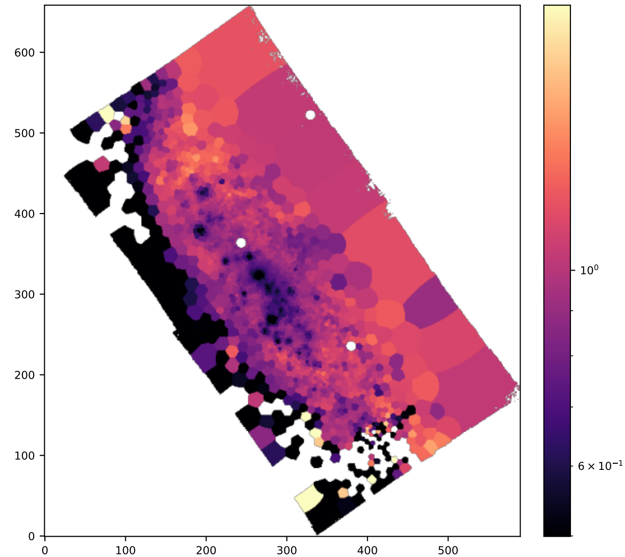
BIN SII/NII
