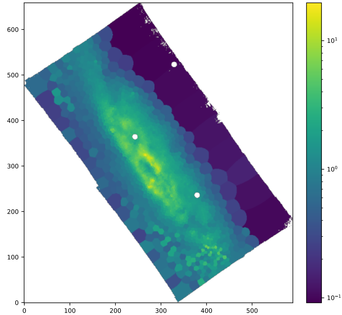
BIN NII6583_SIGMA_ERR
