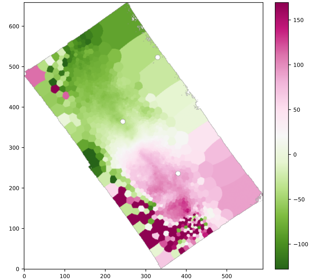
BIN NII6583_VEL
