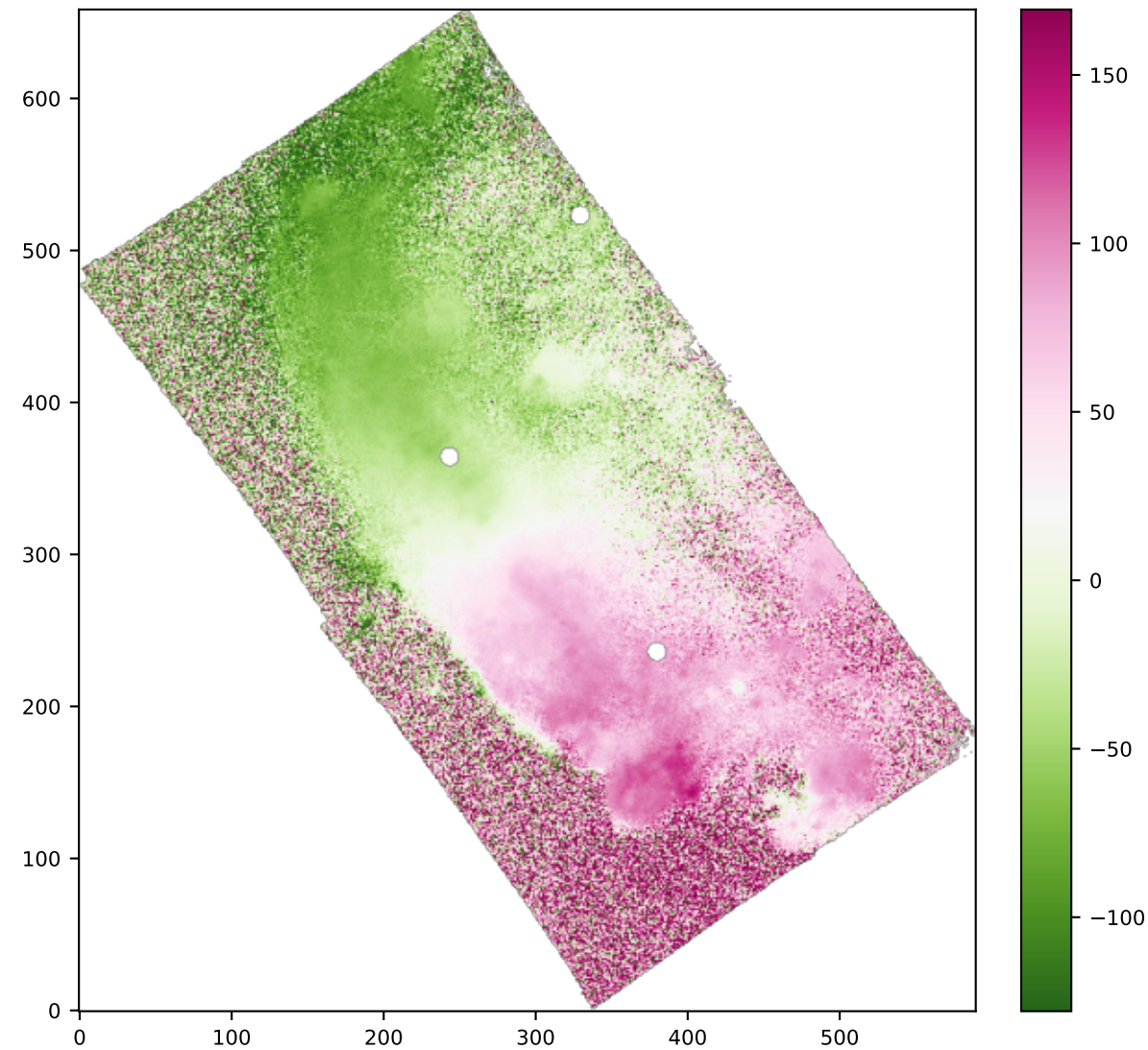
SPAXELS SII6716_VEL
