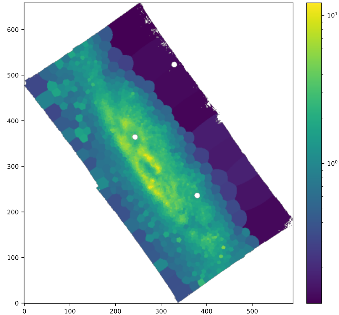
BIN OIII5006_SIGMA_ERR
