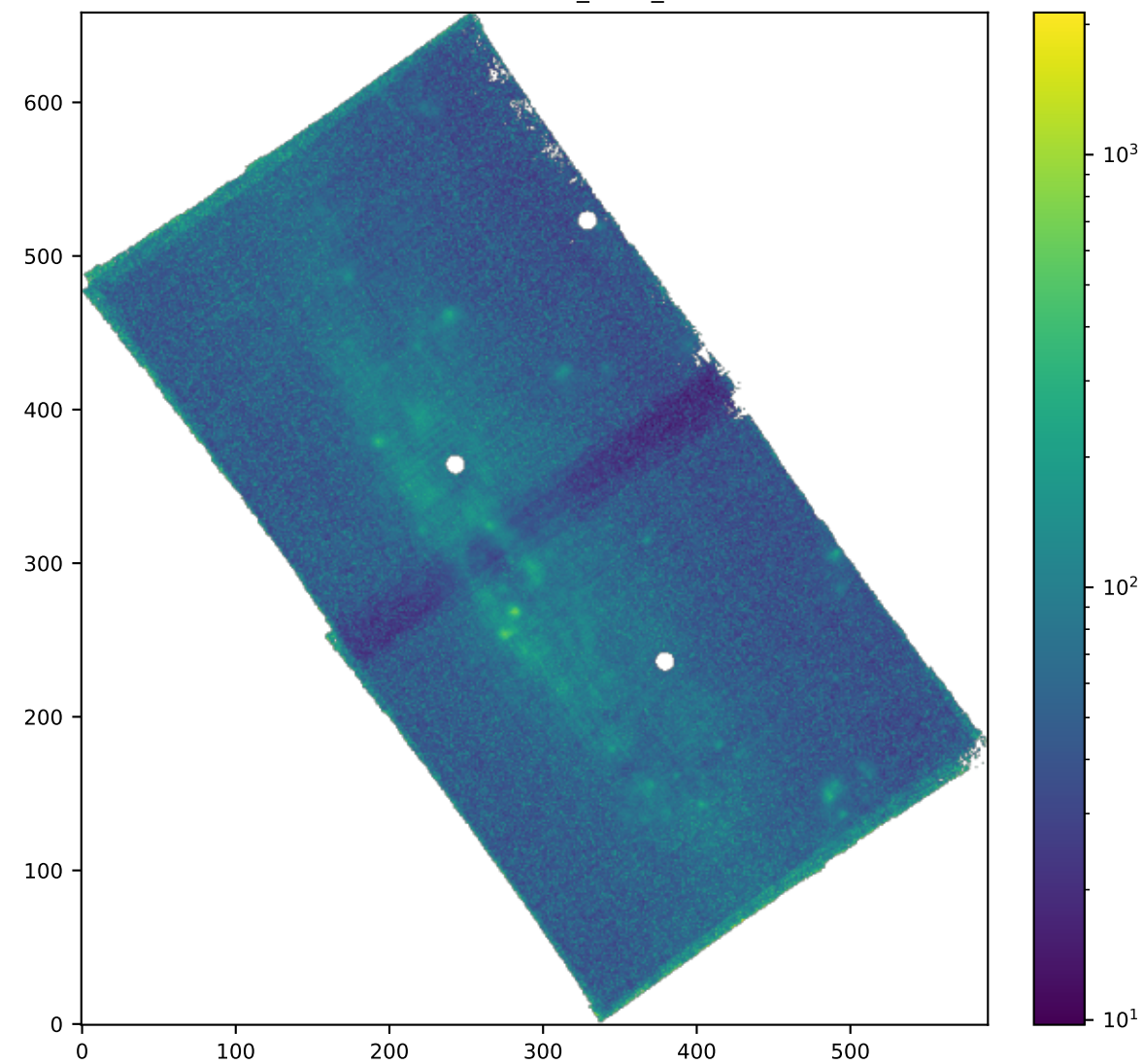
SPAXELS OIII5006_SIGMA_ERR
