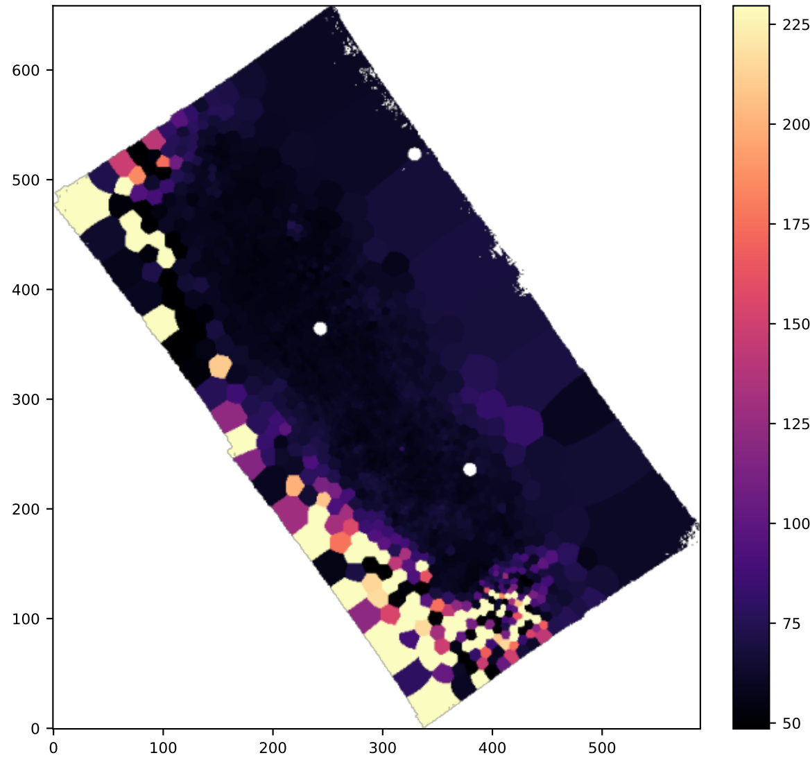
BIN NII6583_SIGMA
