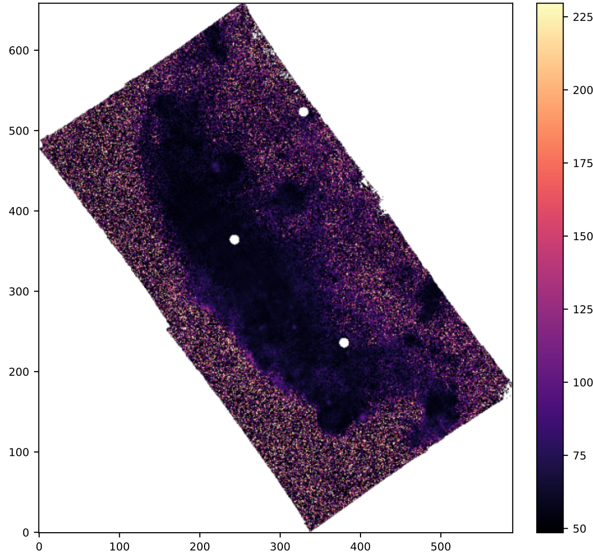
SPAXELS NII6583_SIGMA
