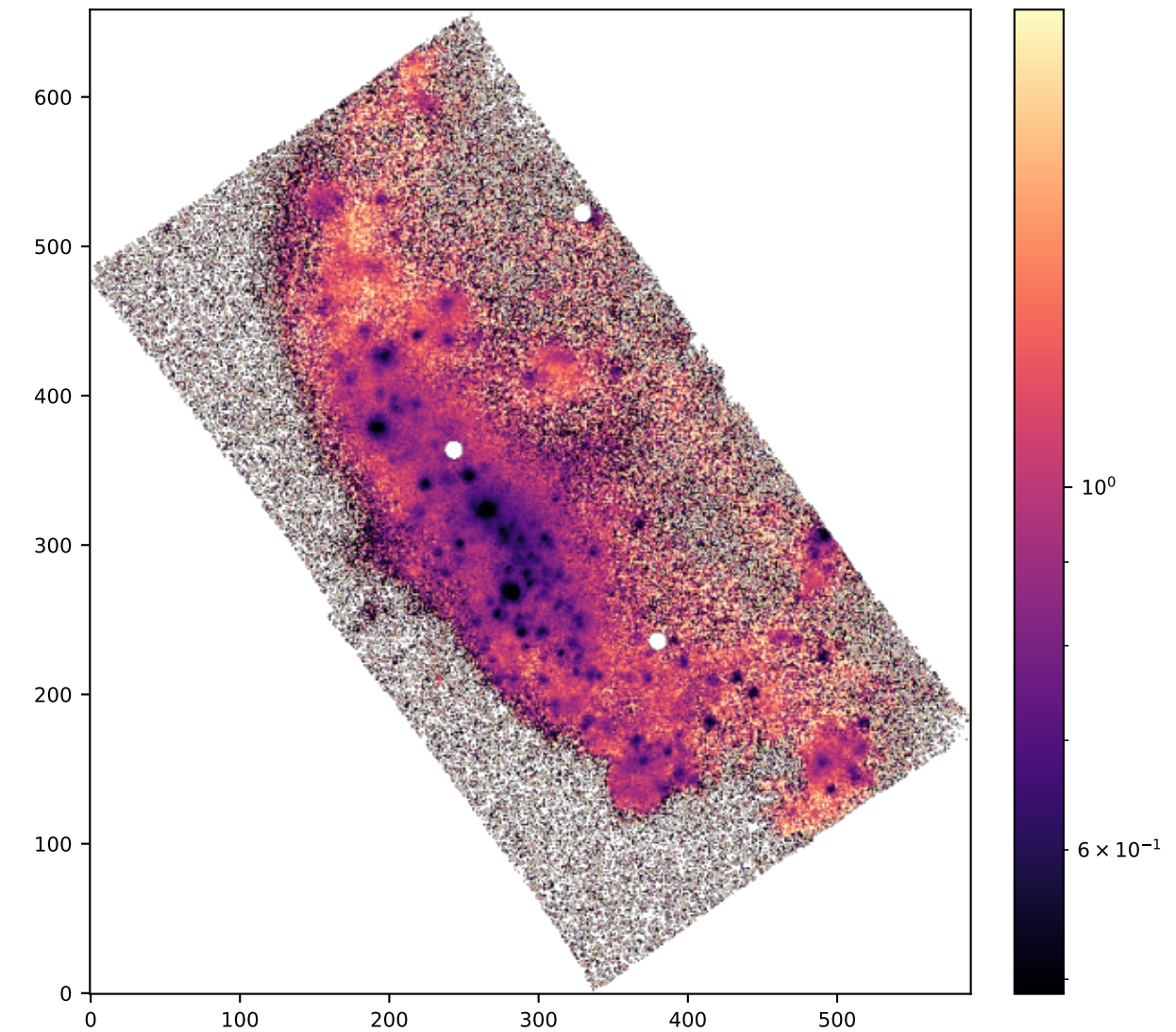
SPAXELS SII/NII
