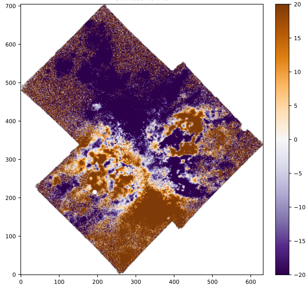
SPAXELS VHa-VNII
