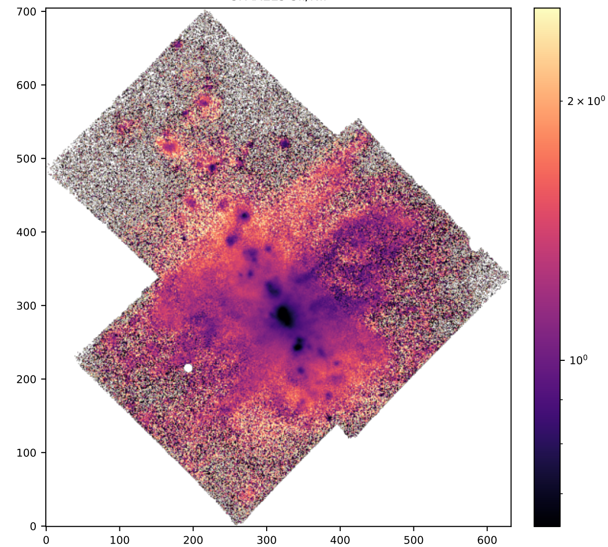
SPAXELS SII/NII
