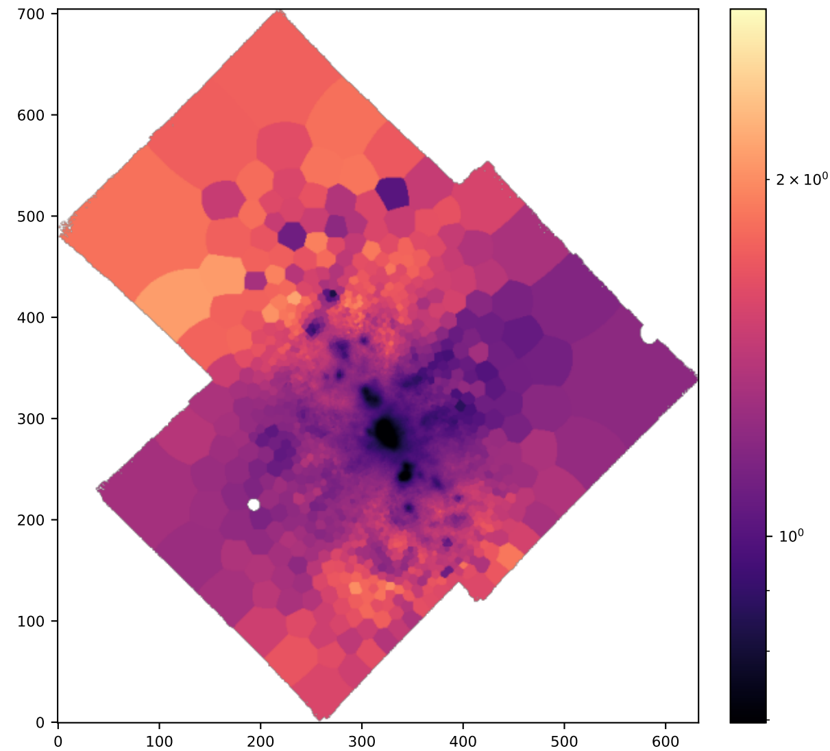
BIN SII/NII
