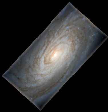
NGC4501
