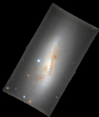
NGC4064
