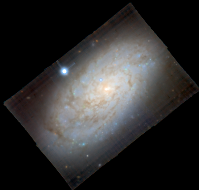
NGC4298
