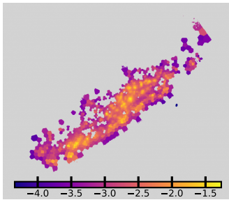
\log \Sigma_{\text{SFR}} (HII)
