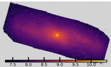
NGC4293: \log \Sigma_*
