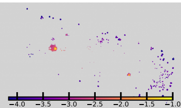
\log \Sigma_{\text{SFR}} (HII)
