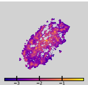
\log \Sigma_{\text{SFR}} (HII)
