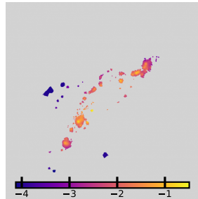
\log \Sigma_{\text{SFR}} (HII)
