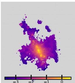
\log \Sigma_{\text{SFR}} (HII)
