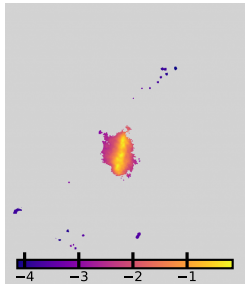
\log \Sigma_{\text{SFR}} (HII)
