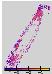
\log \Sigma_{\text{SFR}} (HII)
