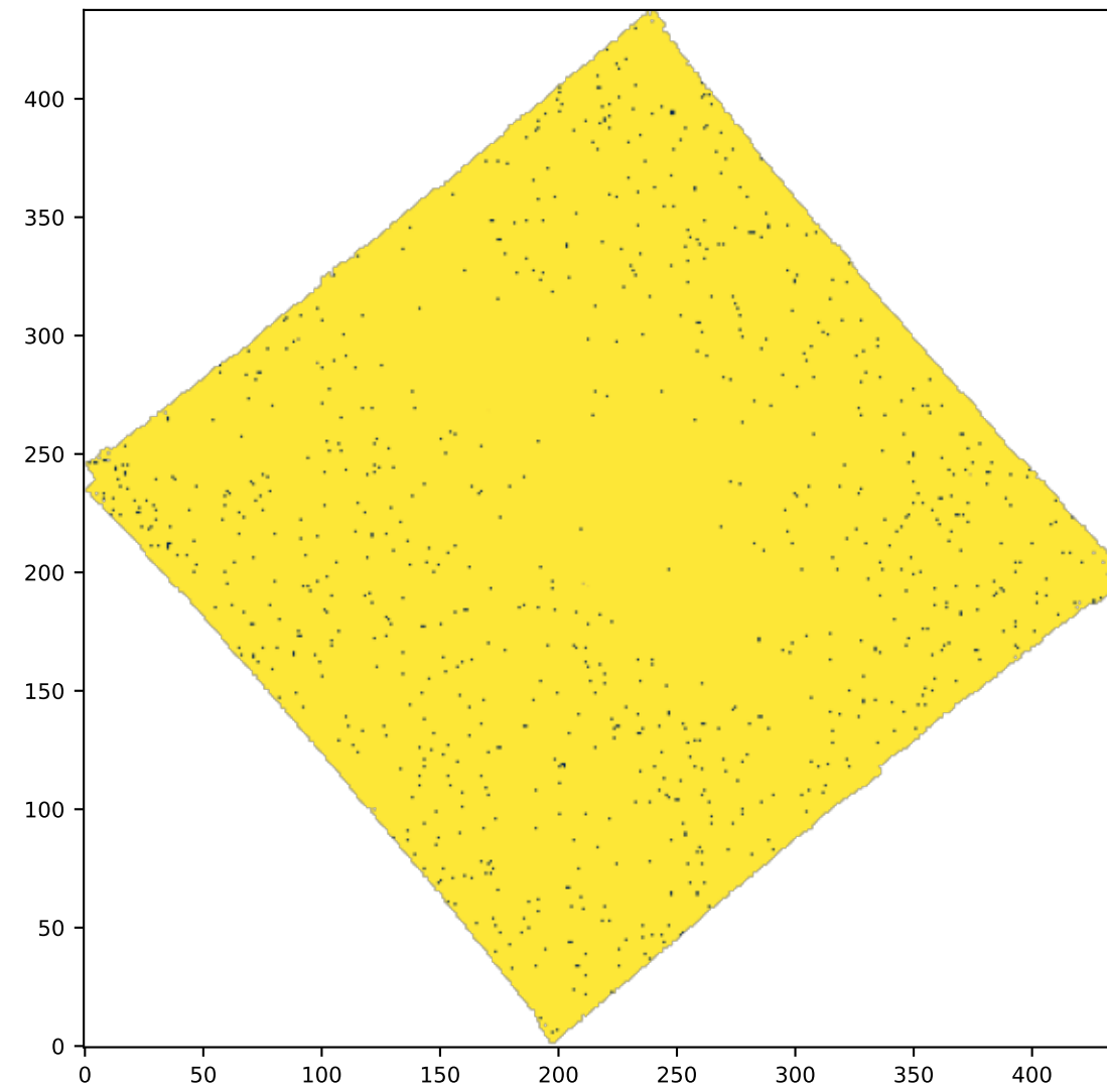
SPAXELS OIII5006_SIGMA_ERR
