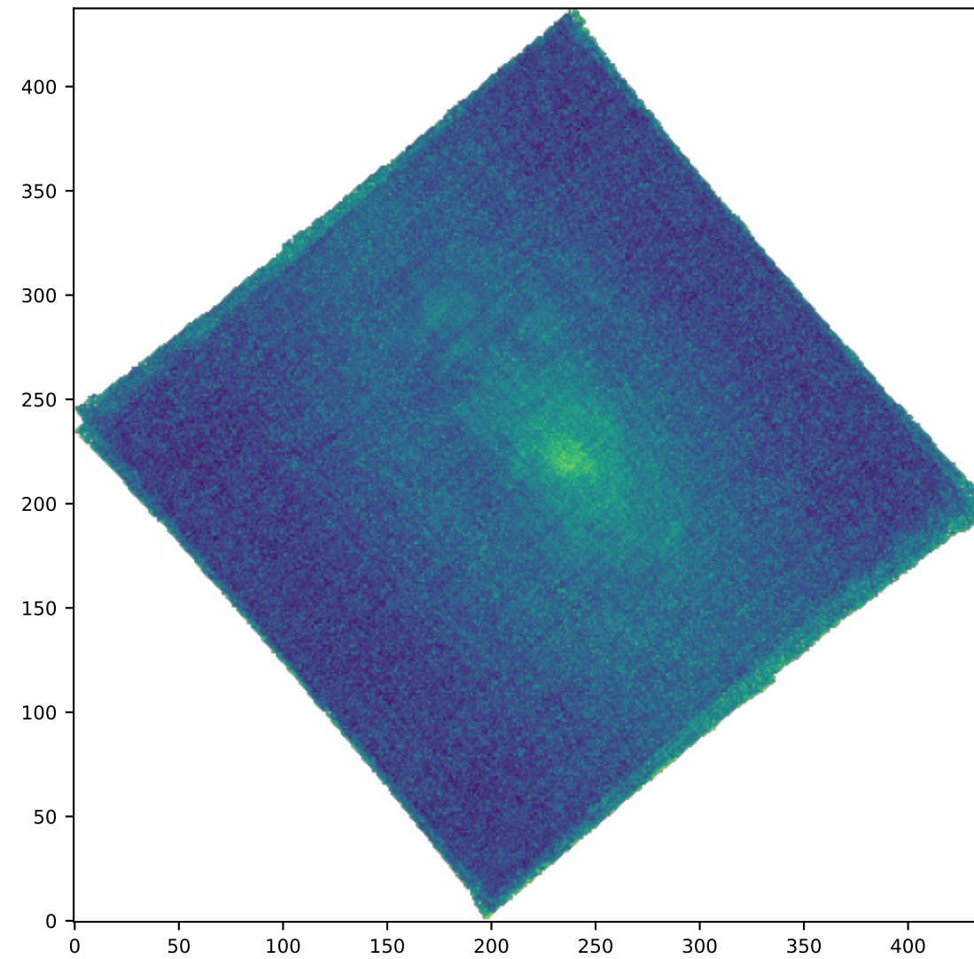
SPAXELS OIII5006_SIGMA_ERR
