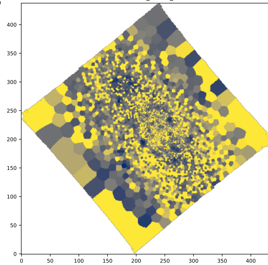
BIN OIII5006_SIGMA_ERR
