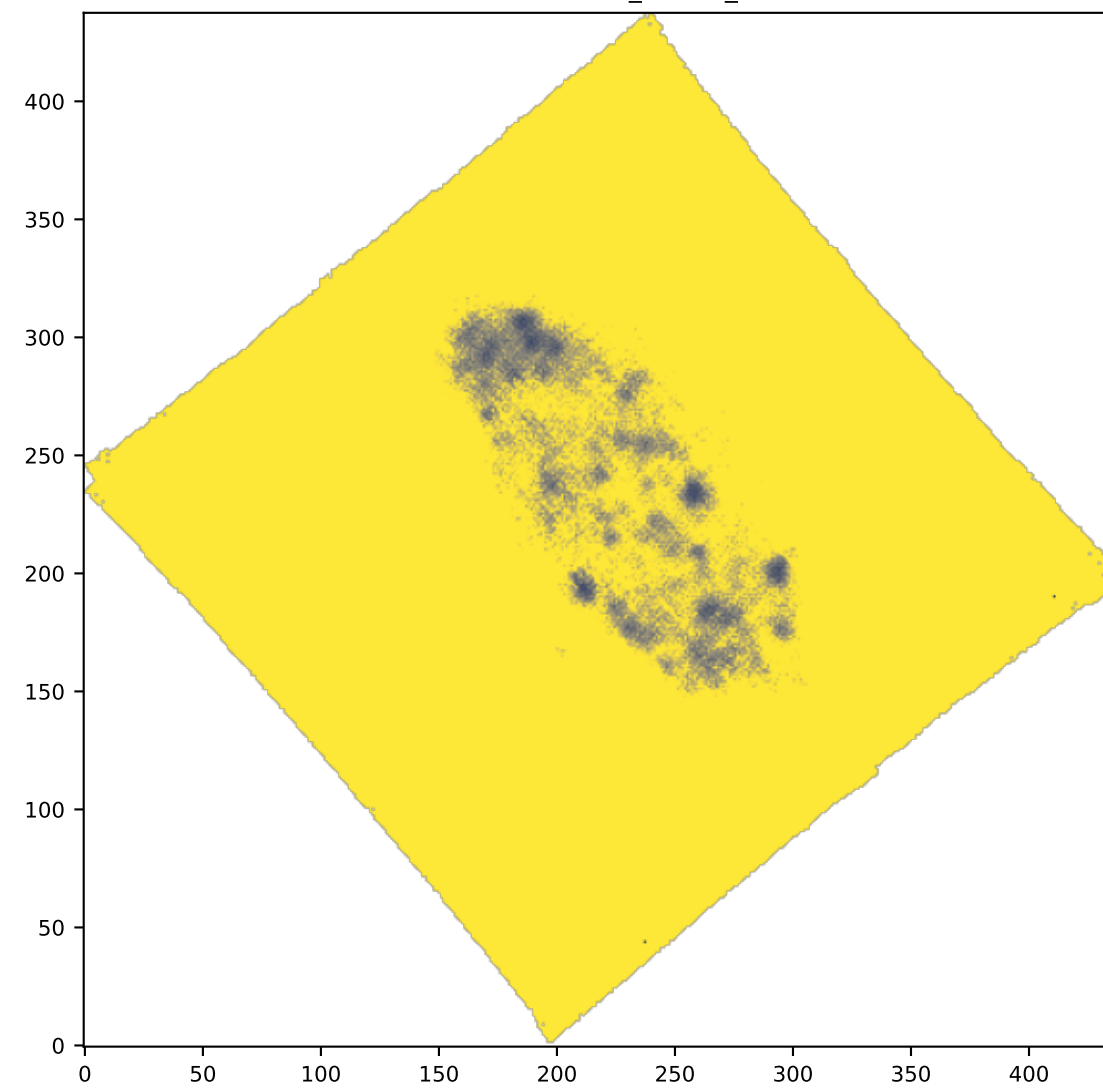
SPAXELS NII6583_SIGMA_ERR
