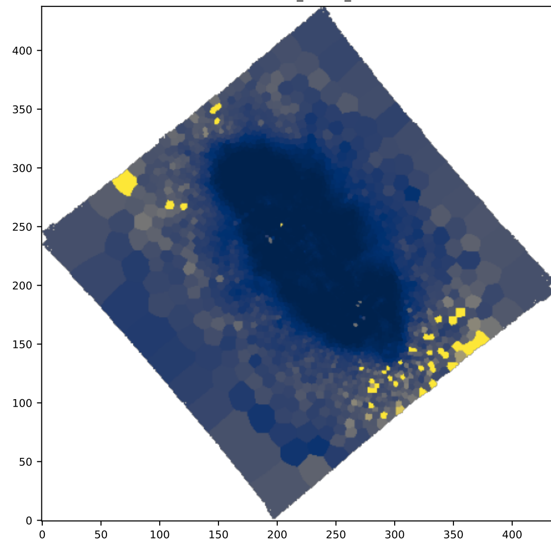
BIN HA6562_SIGMA_ERR
