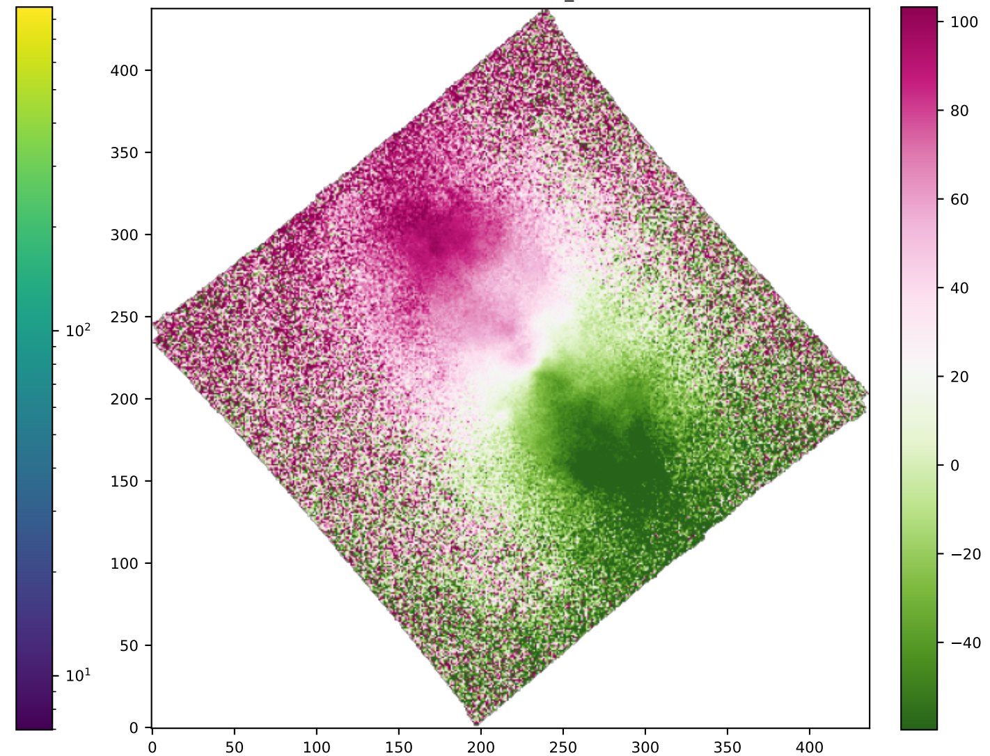
SPAXELS SII6716_VEL
