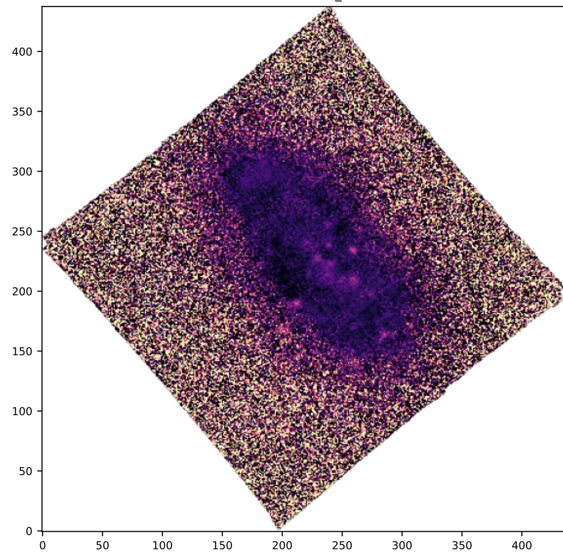
SPAXELS NII6583_SIGMA
