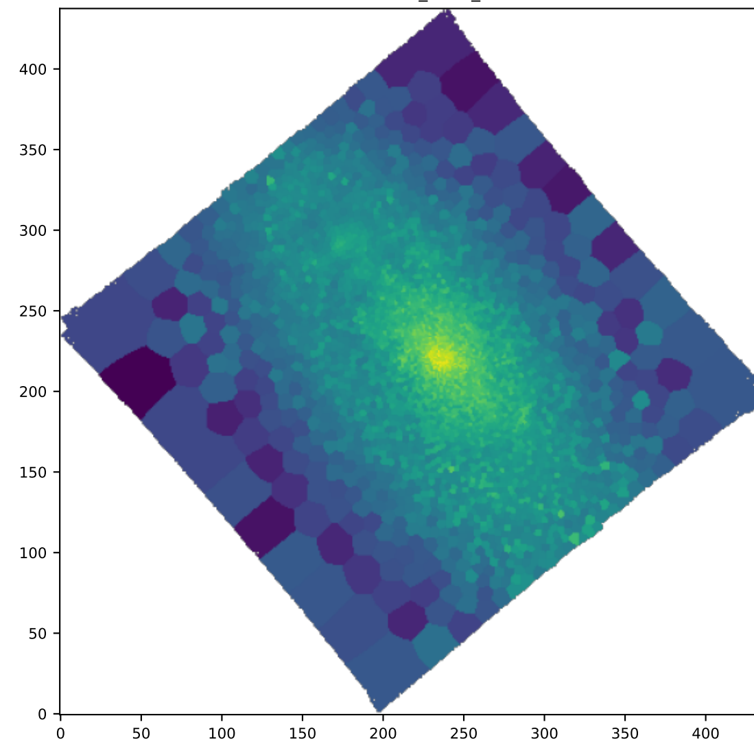
BIN OIII5006_SIGMA_ERR
