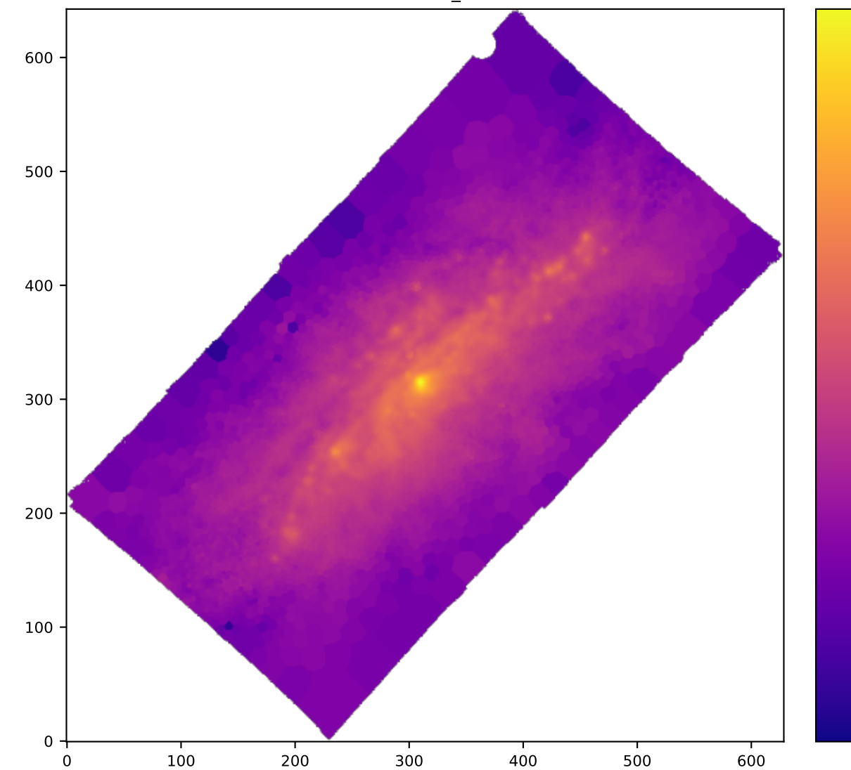
BIN NII6583_SIGMA
