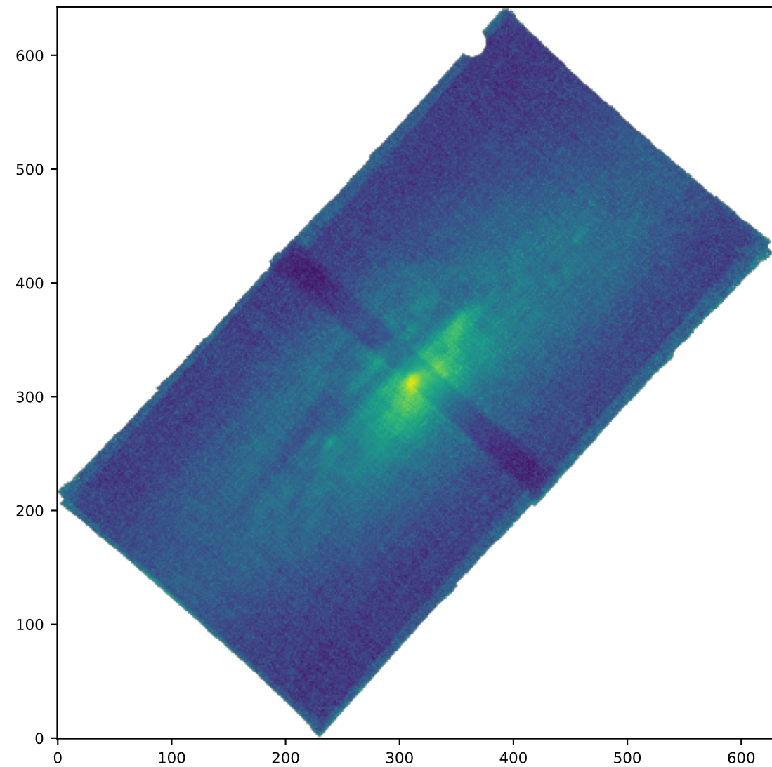
SPAXELS OIII5006_SIGMA_ERR
