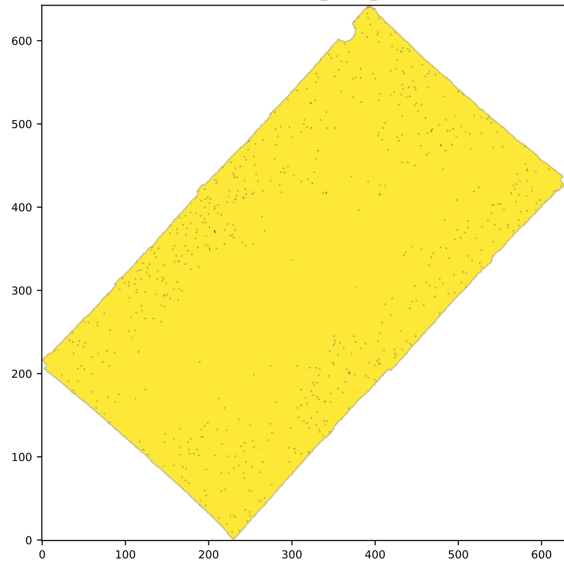
SPAXELS OIII5006_SIGMA_ERR
