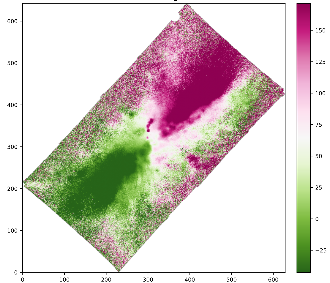
SPAXELS SII6716_VEL
