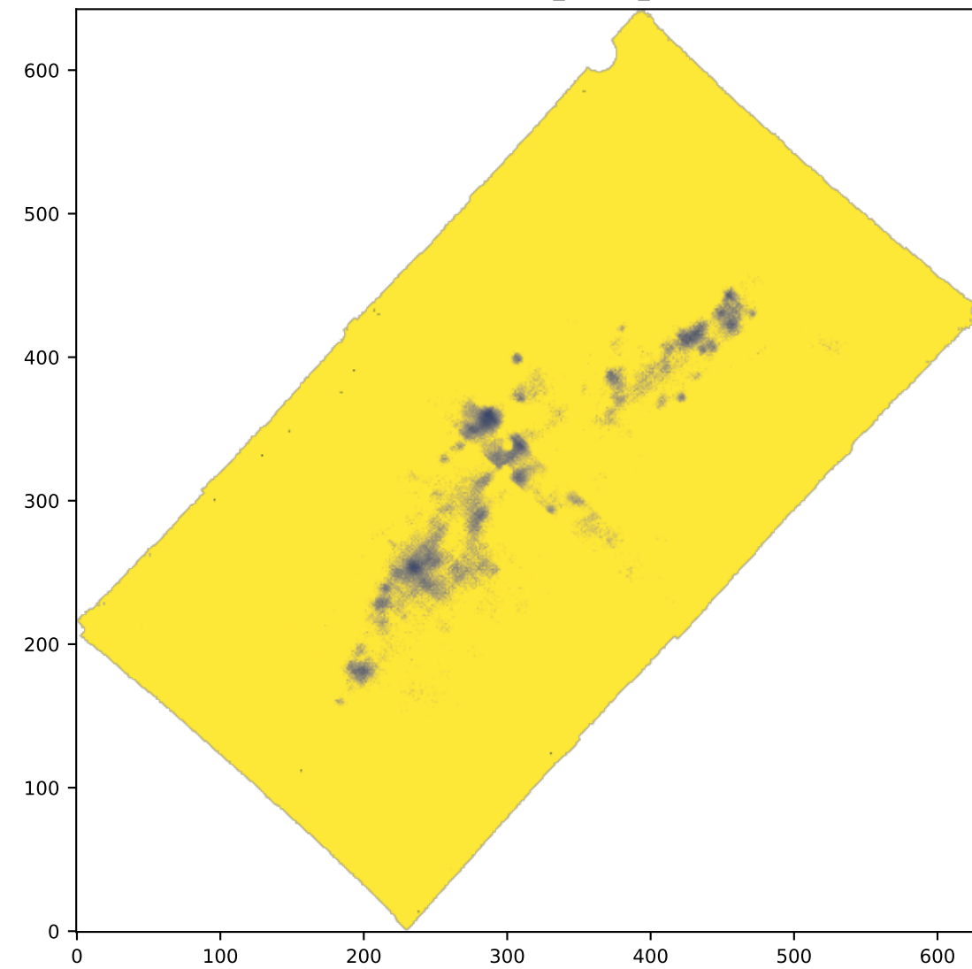
SPAXELS NII6583_SIGMA_ERR
