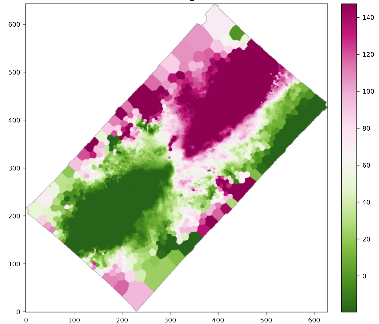
BIN NII6583_VEL
