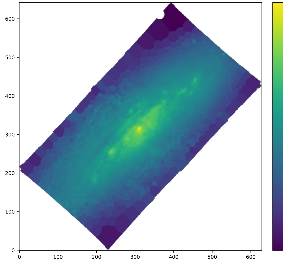
BIN HA6562_SIGMA_ERR
