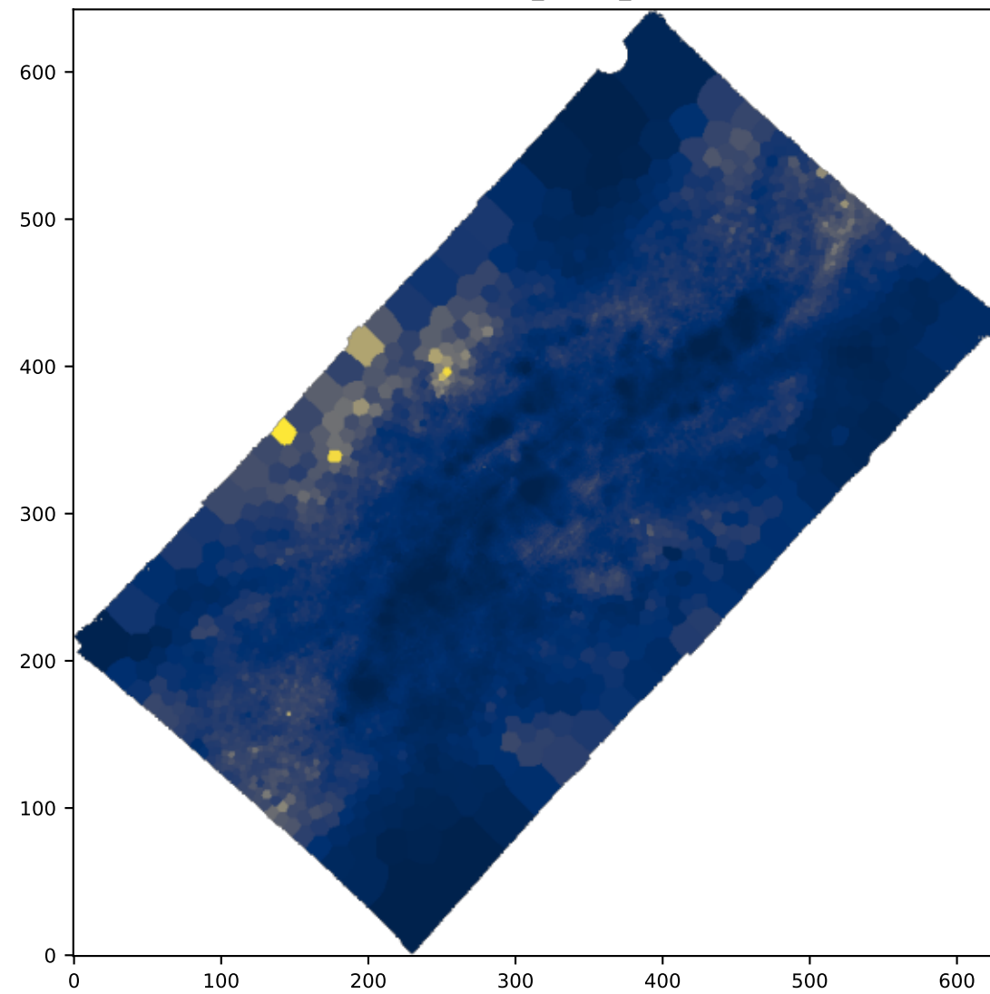
BIN NII6583_SIGMA_ERR
