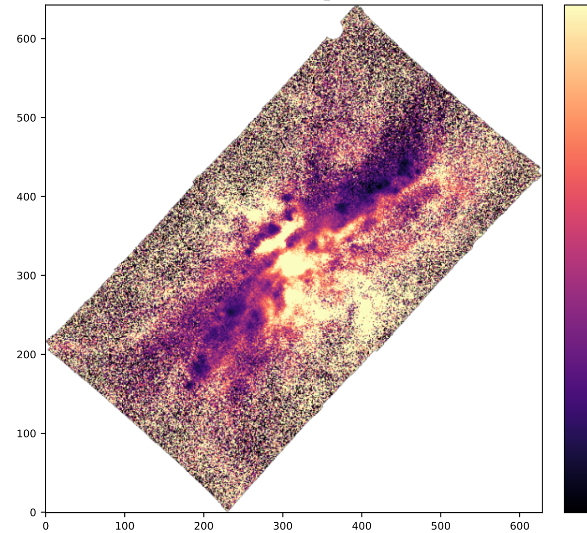
SPAXELS NII6583_SIGMA
