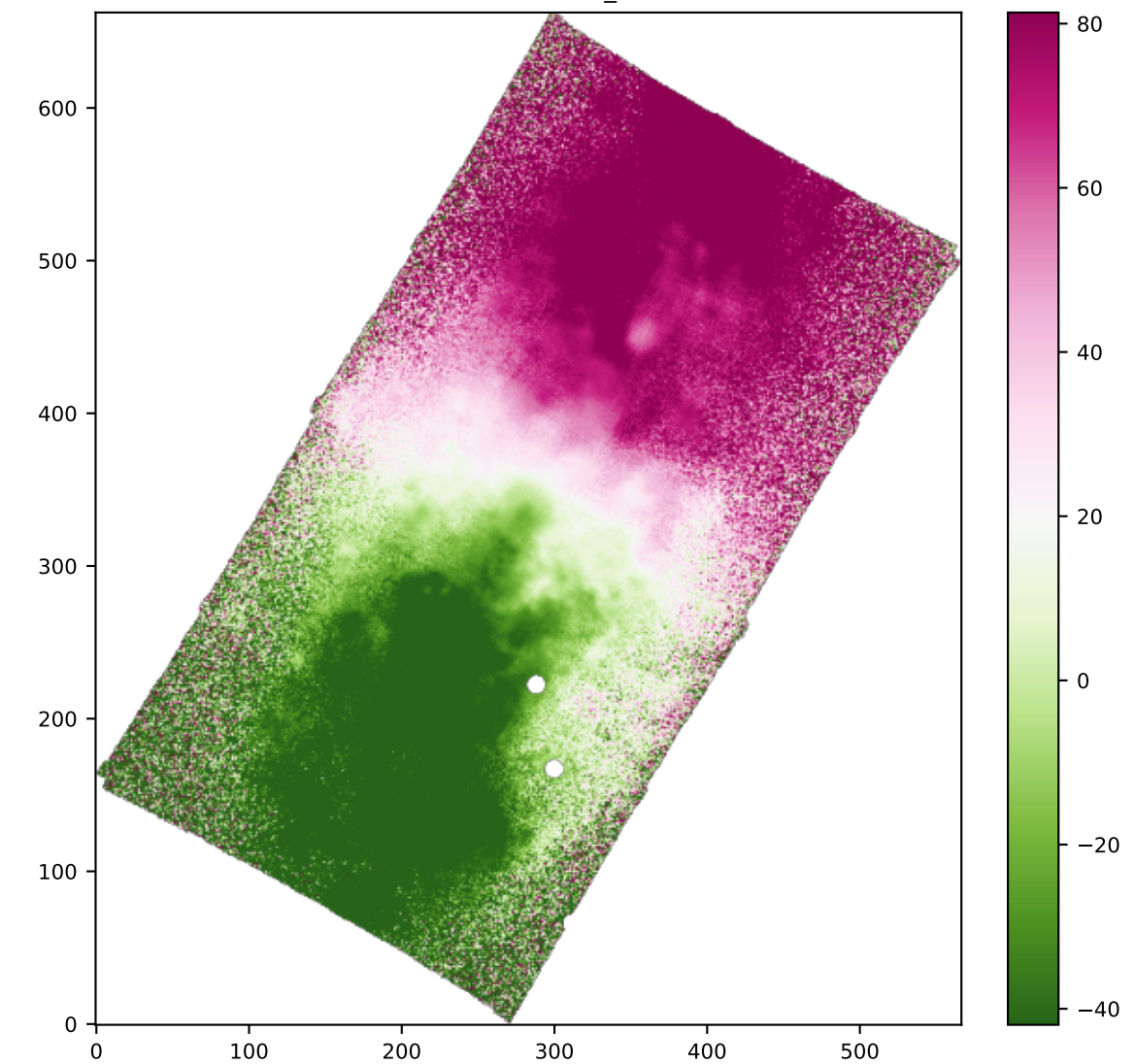
SPAXELS SII6716_VEL
