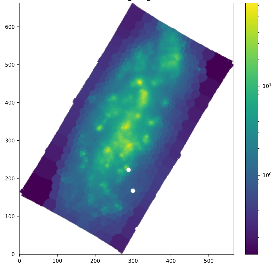
BIN HA6562_SIGMA_ERR
