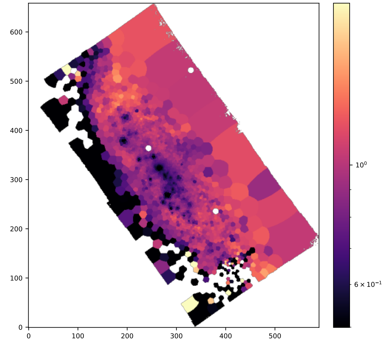
BIN SII/NII
