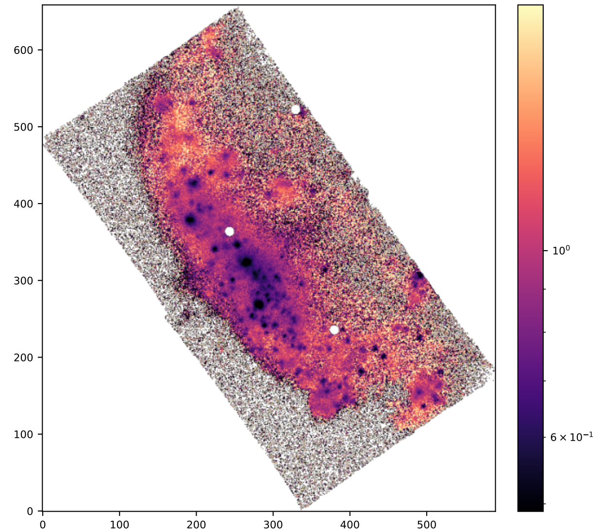
SPAXELS SII/NII
