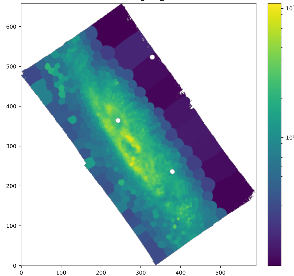
BIN OIII5006_SIGMA_ERR
