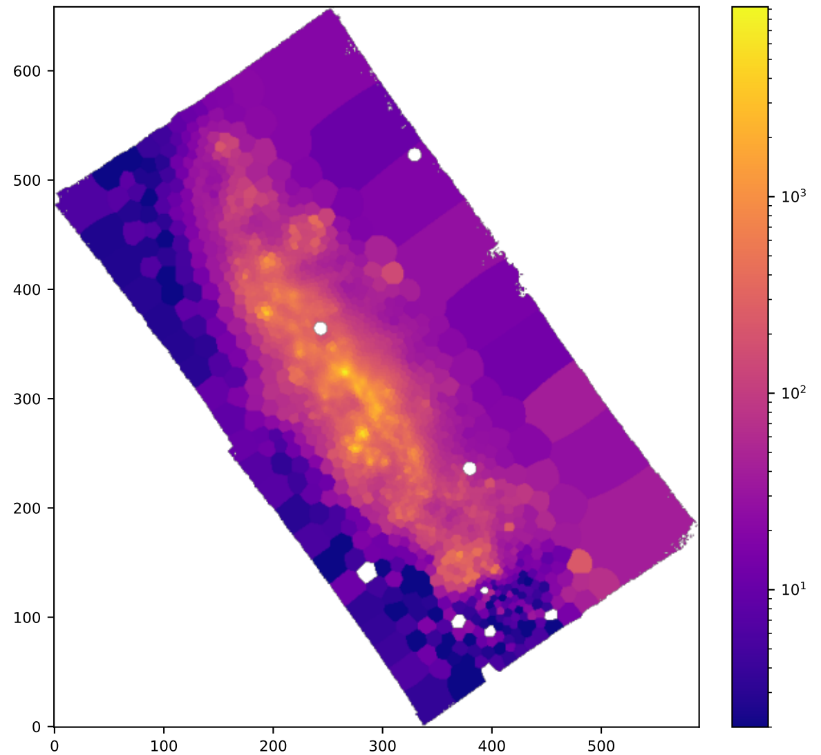
BIN NII6583_SIGMA
