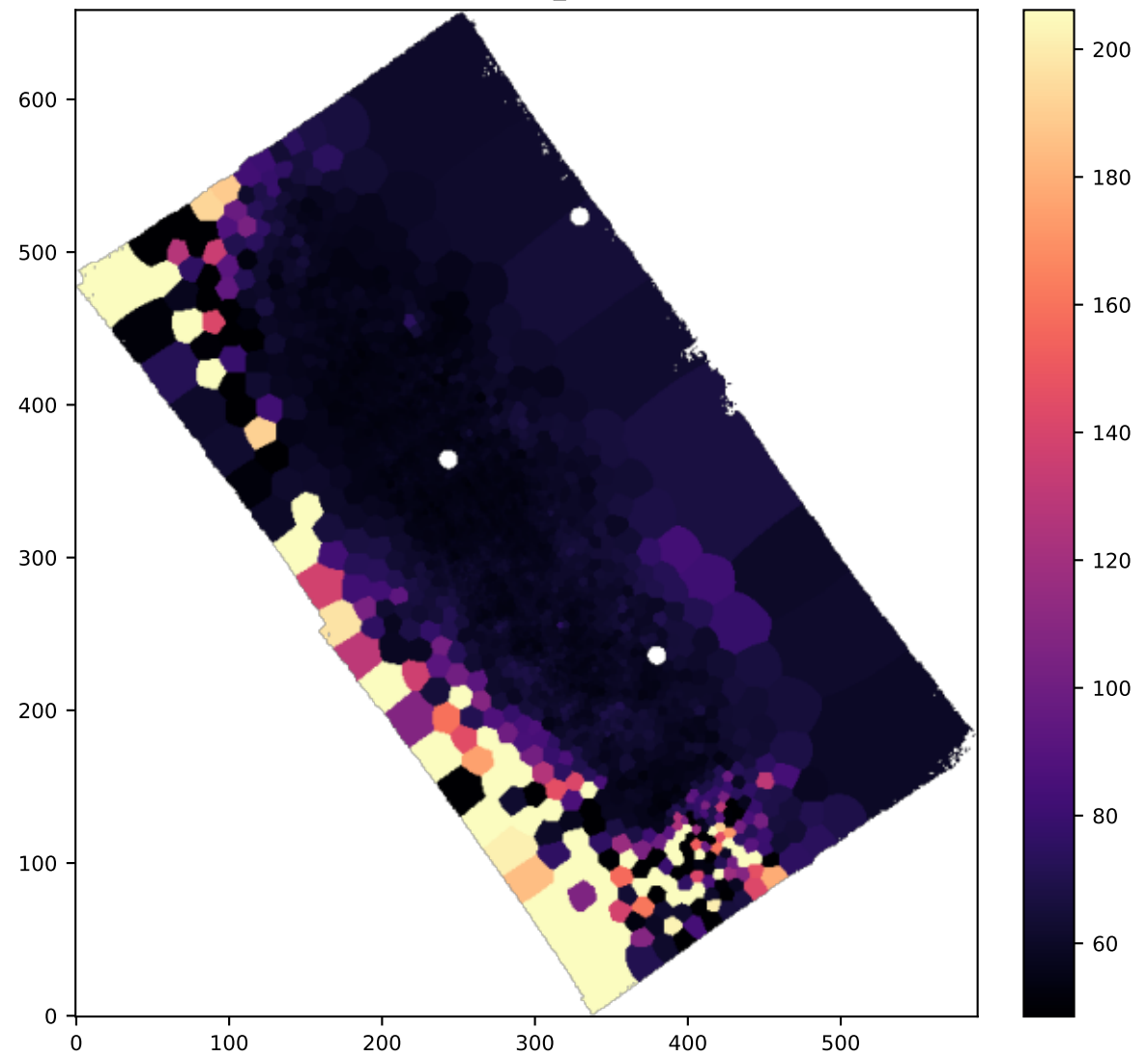
BIN NII6583_SIGMA
