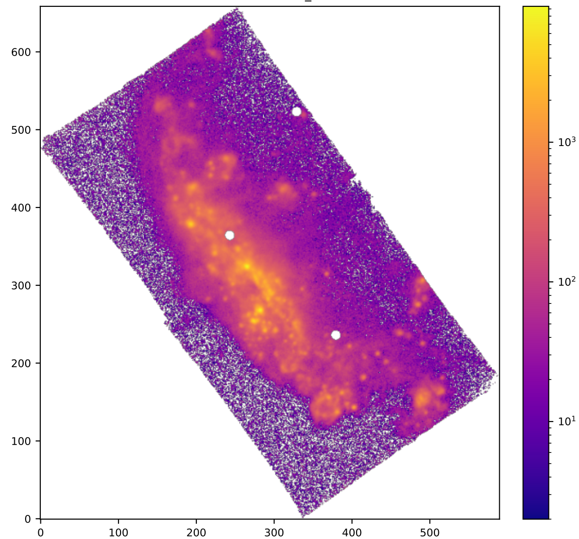
SPAXELS NII6583_SIGMA
