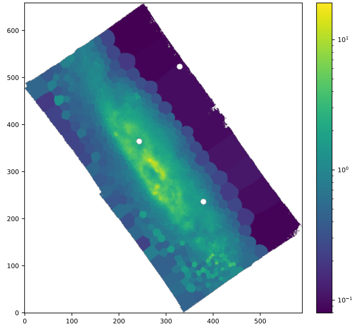
BIN NII6583_SIGMA_ERR
