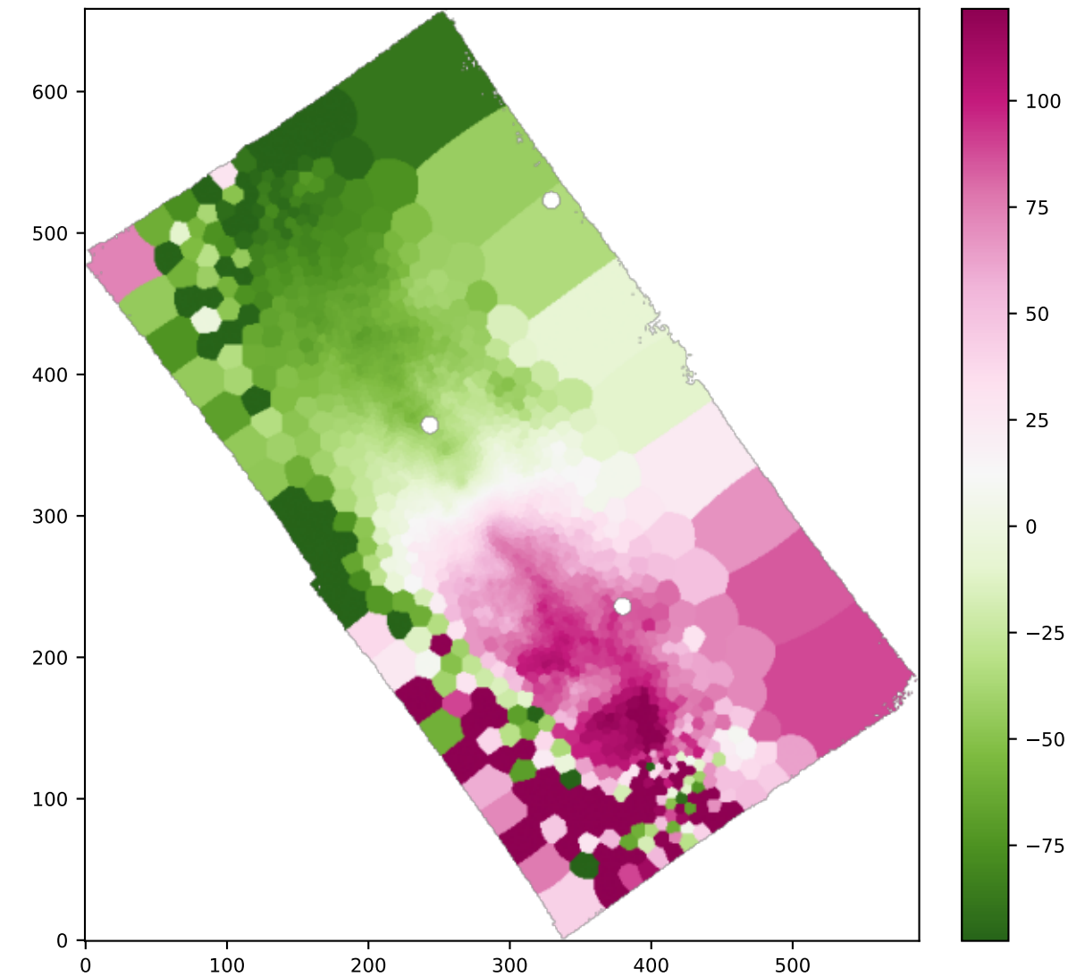
BIN NII6583_VEL
