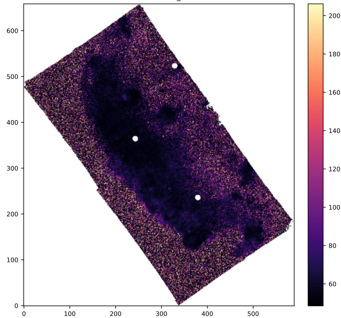
SPAXELS NII6583_SIGMA
