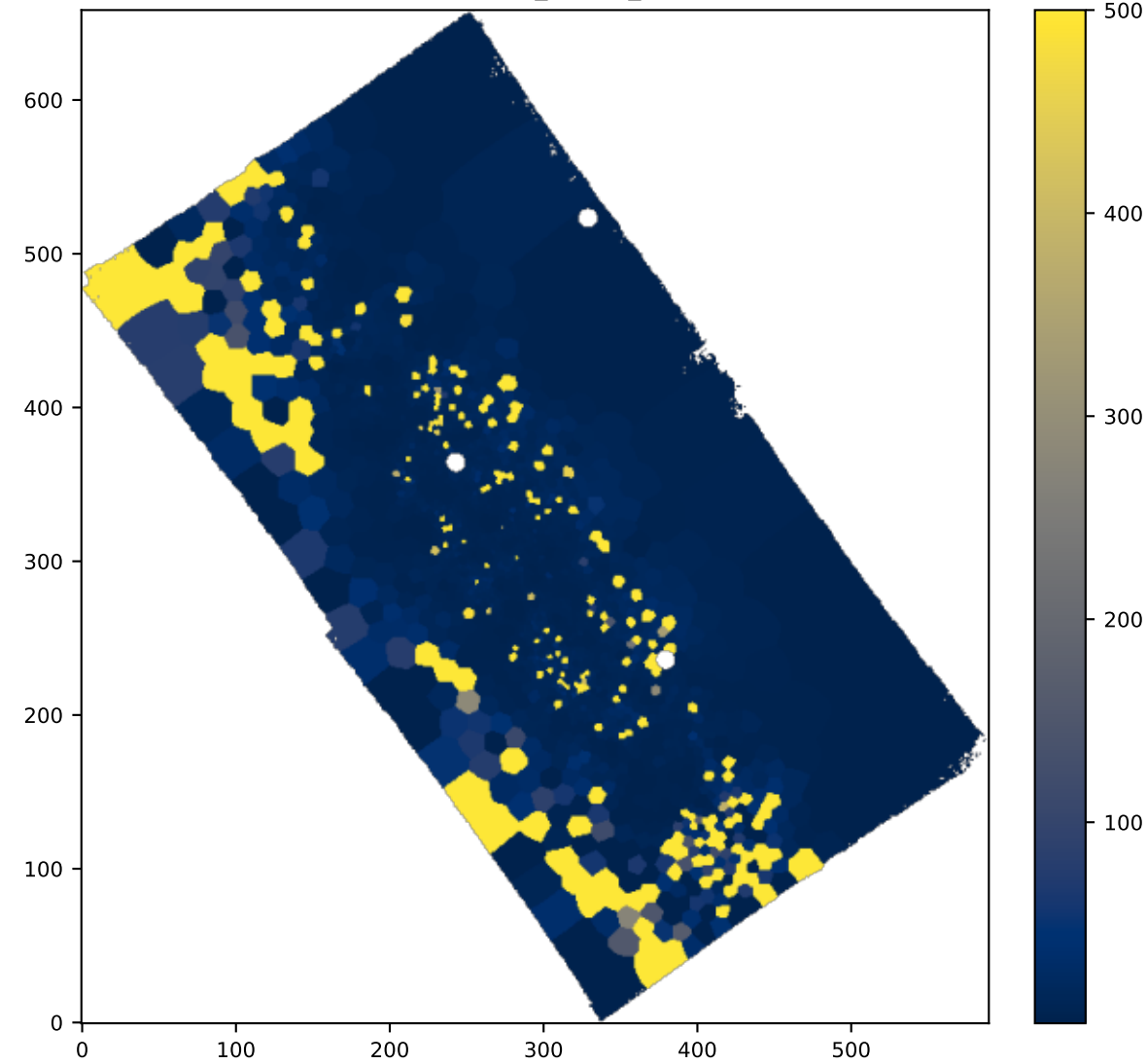
BIN OIII5006_SIGMA_ERR
