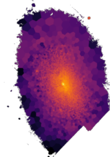
NGC4501
