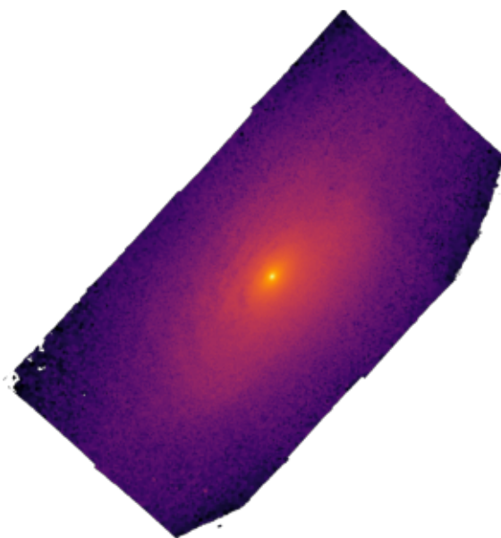
NGC4501
