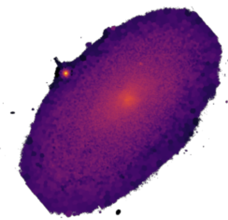
NGC4298
