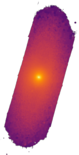
NGC4698
