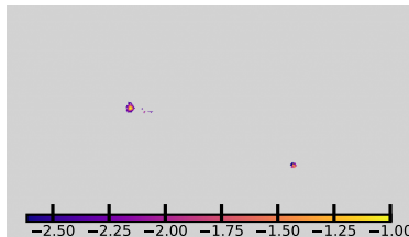
\log \Sigma_{\text{SFR}} (HII)
