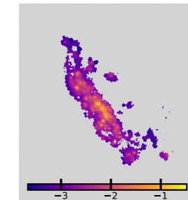
\log \Sigma_{\text{SFR}} (HII)
