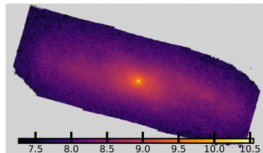
NGC4293: \log \Sigma_*
