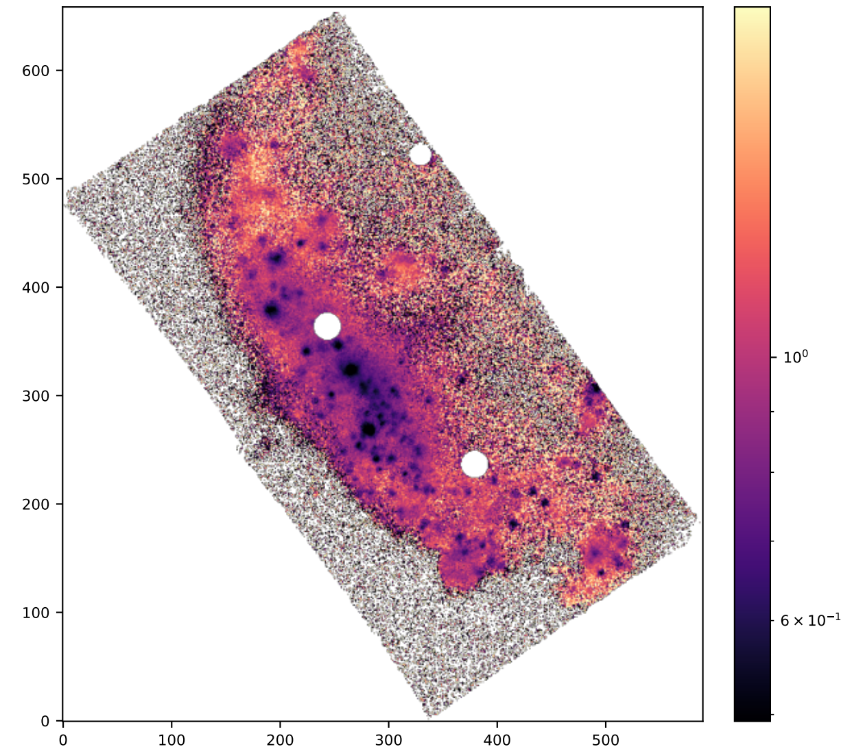
SPAXELS SII/NII
