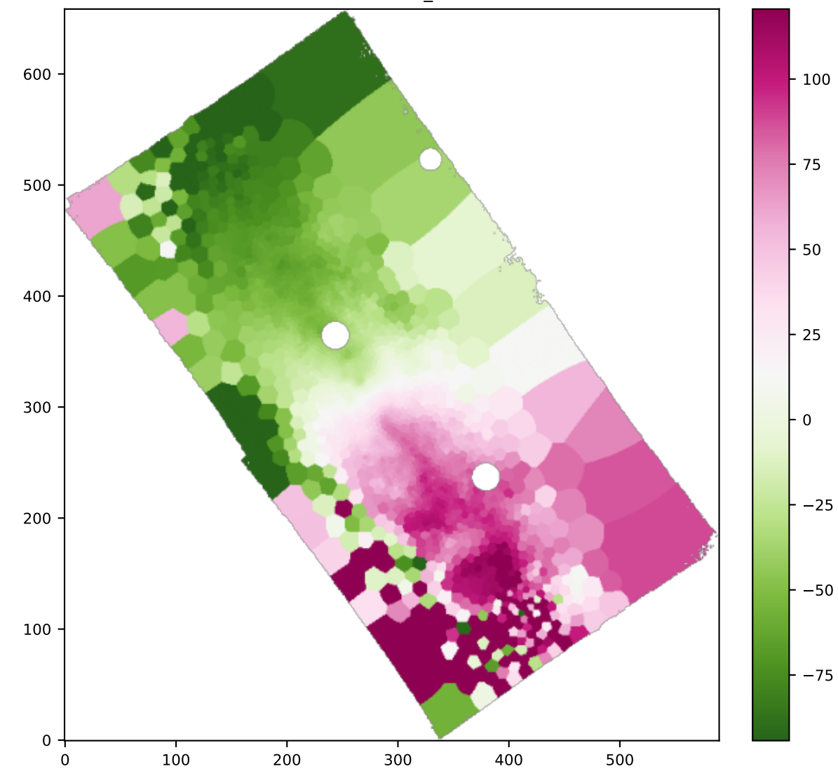
BIN NII6583_VEL
