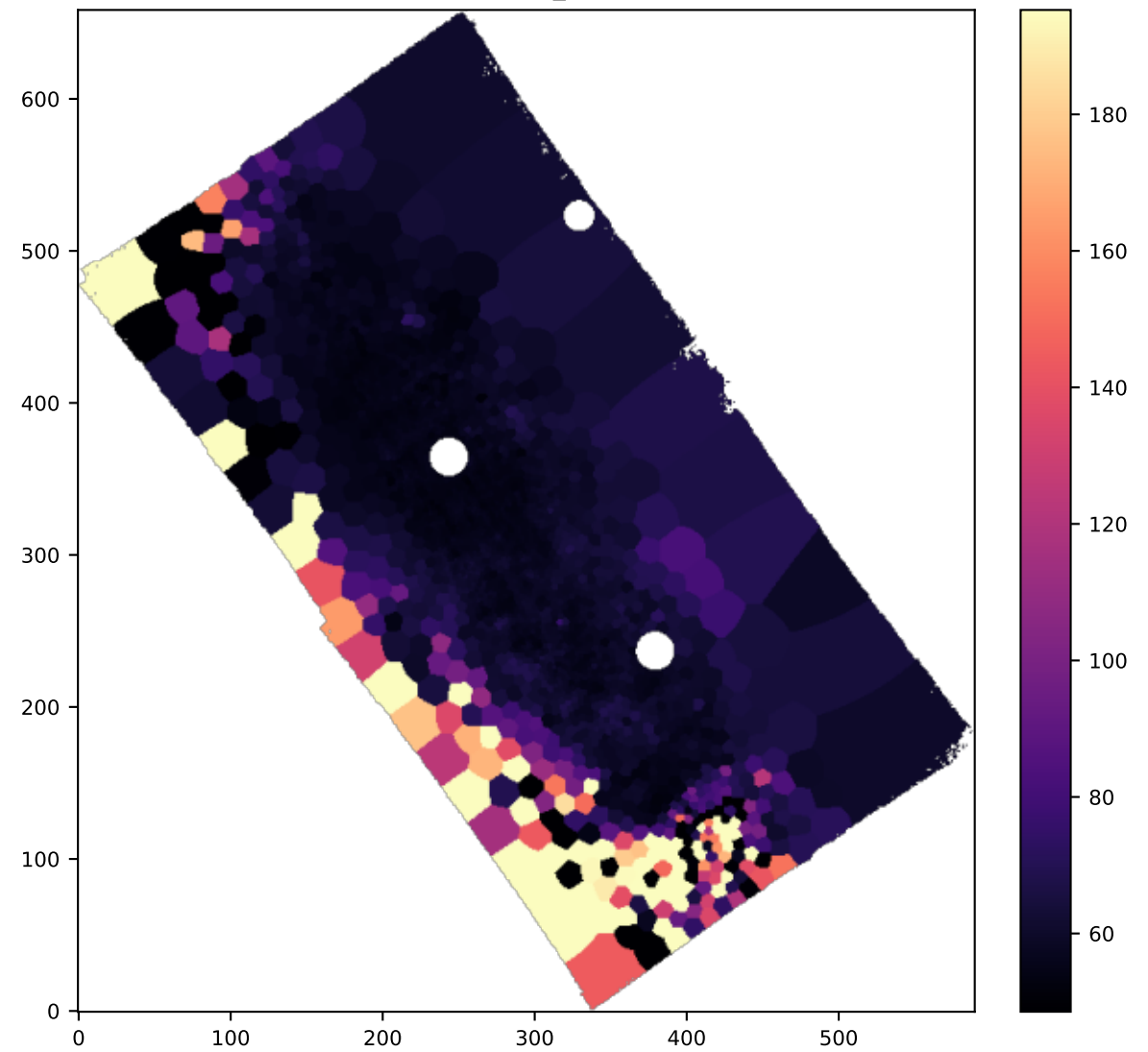
BIN NII6583_SIGMA
