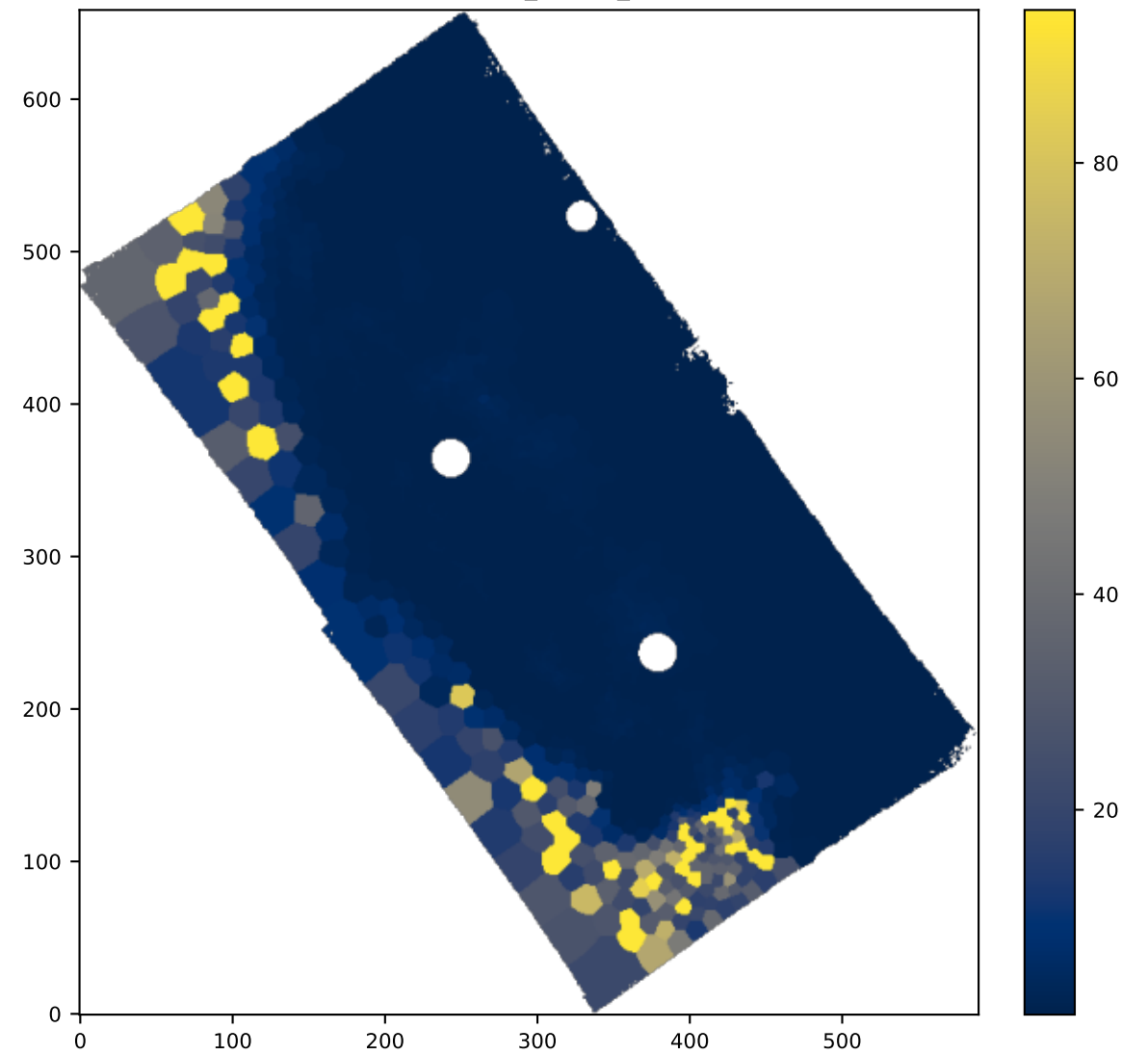
BIN NII6583_SIGMA_ERR
