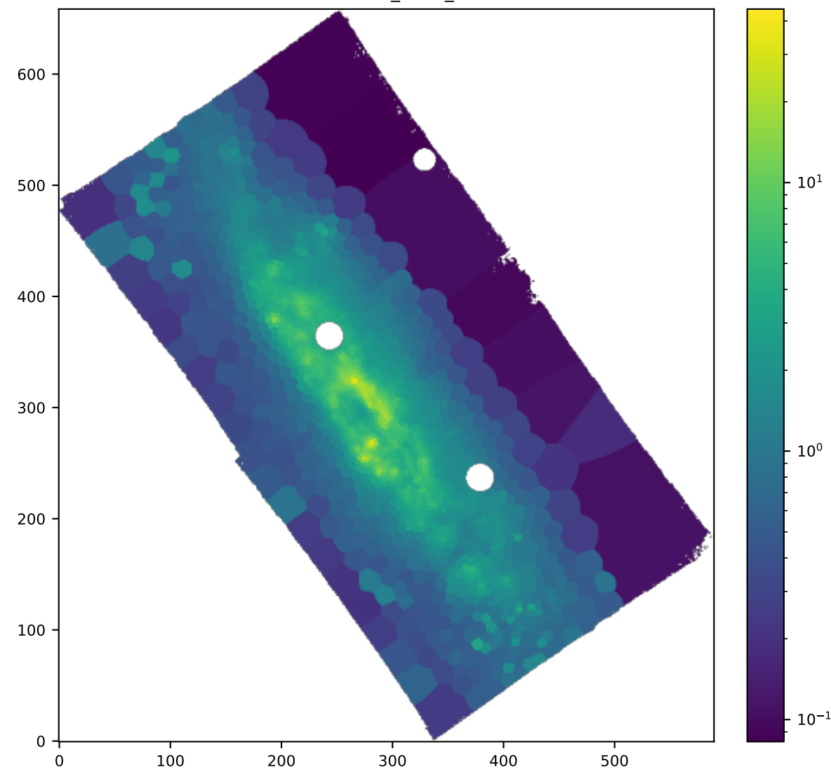
BIN HA6562_SIGMA_ERR
