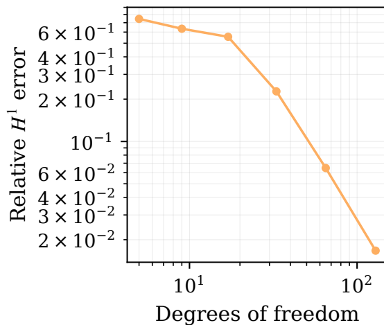
Pure p=4 , d=2
