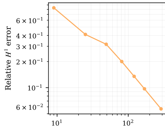
Sinh, d=2
