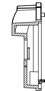
SECTION A-A SCALE 1 : 1.5
