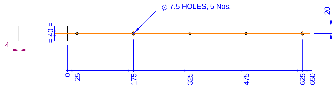
GASKET 3 - BASE FRAME (QTY : 2 Nos.) MATERIAL : GIVEN
