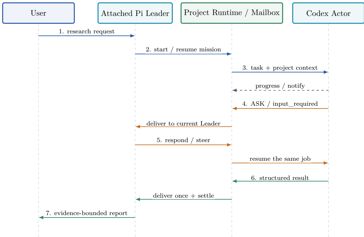
图 2: Codex 消息先进入 Project Runtime，再交给当前 attached Leader。蓝色 1-3 是任务路径，橙色 4-5 是阻塞 ASK 往返，绿色 6-7 是结果路径；灰色虚线 progress 只供 /watch 观察。ASK 通过精确的 job ID 和 request ID 返回同一 Codex turn；Session 轮换只改变 Leader attachment，不改变 Action、mailbox 和 mission 的 Project 归属。
