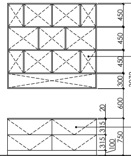
CATALOG SHELF ELEVATION
