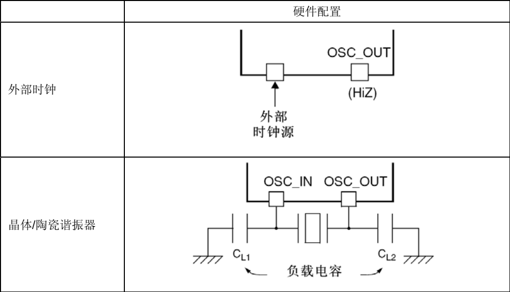
图12 HSE/LSE时钟源
