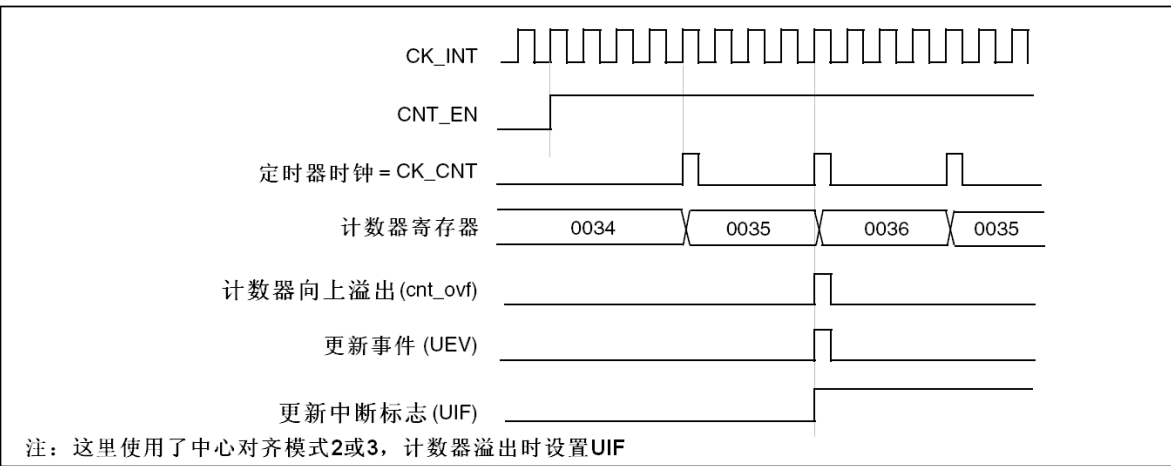
图114 计数器时序图，内部时钟分频因子为4，TIMx_ARR=0x36
