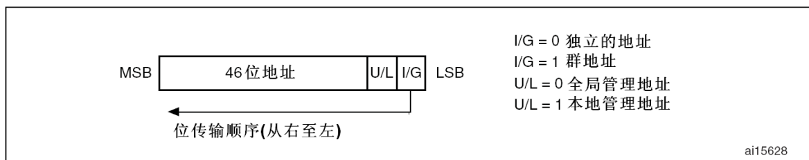
图305 地址域格式
