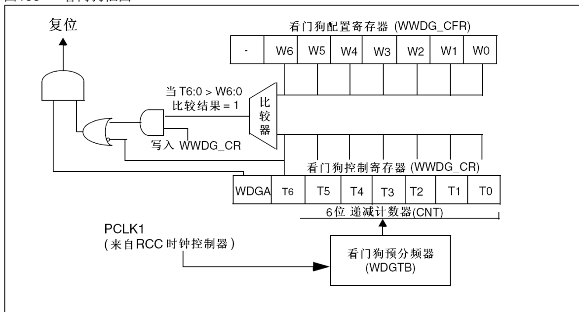
图158 看门狗框图
