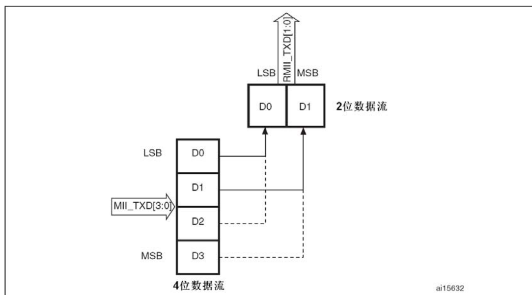
图308 位传输顺序
