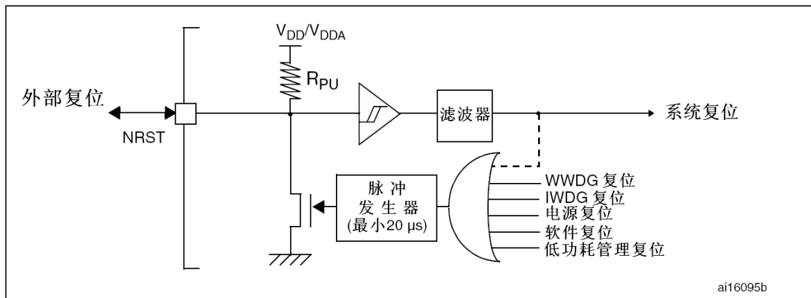
图10 复位电路
