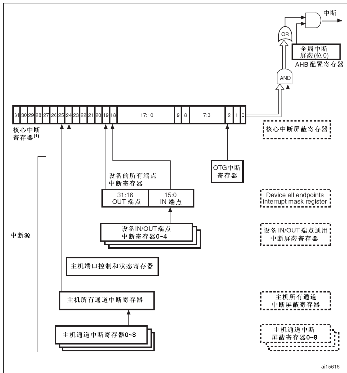
图280 中断架构
