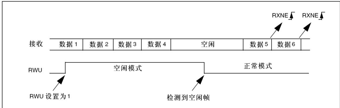
图254 利用空闲总线检测的静默模式
