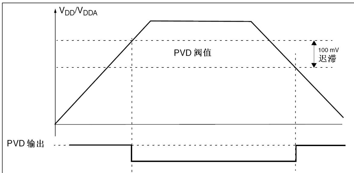
图6 PVD的门限
