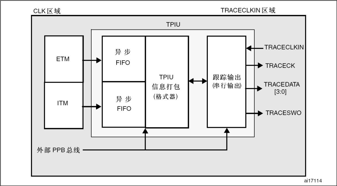
图335 TPIU框图
