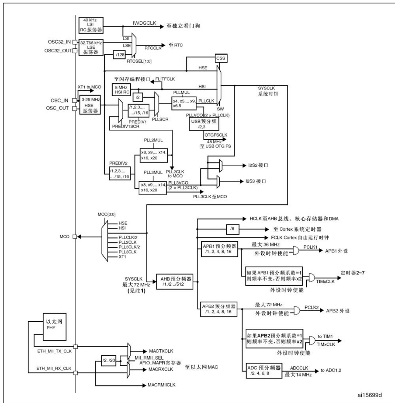
图11 时钟树
