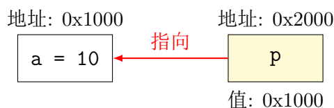
图 4.1: 指针变量 p 指向变量 a 的内存关系图
