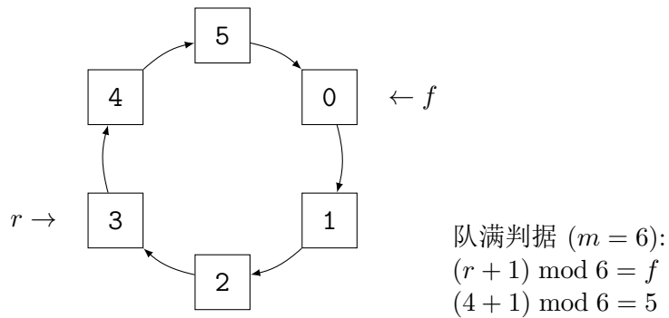
图 3.8: 循环队列 (Circular Queue)
