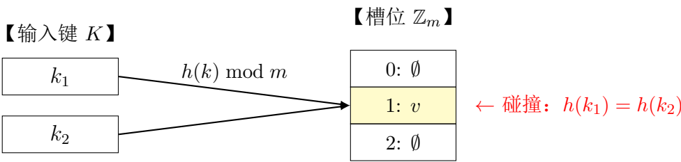
图 3.10: 哈希碰撞三大核心要素模型
