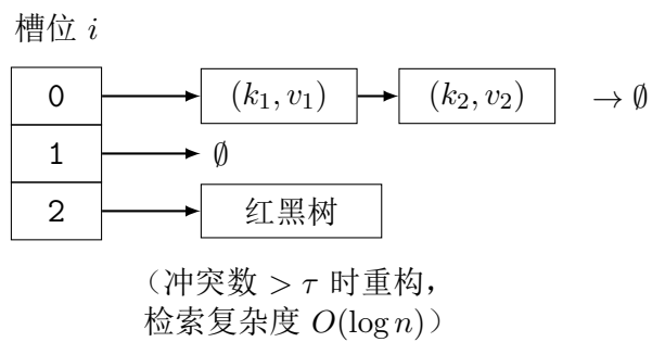
图 3.6: 链地址法与动态重构模型
