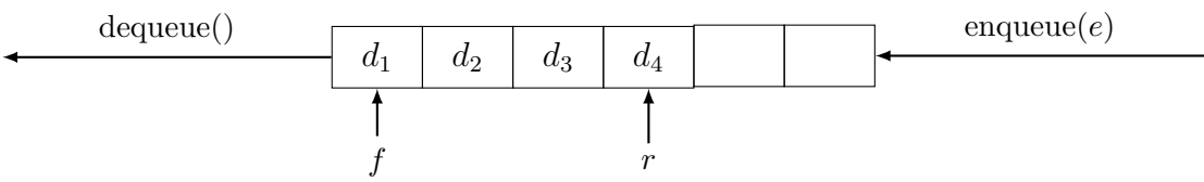
图 3.2: 普通队列 (Queue)
