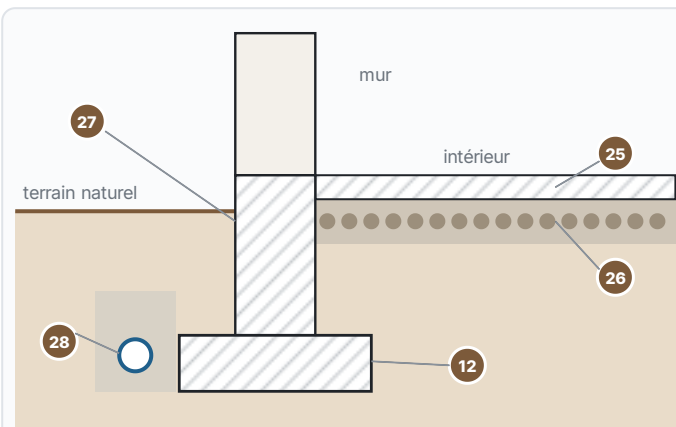
Coupe sur une fondation (semelle filante).
