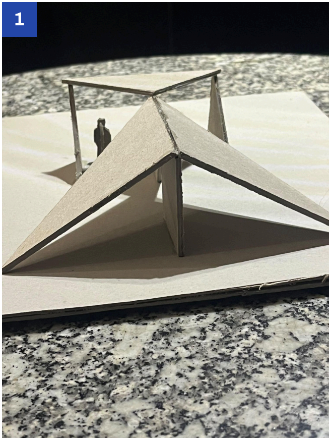
Le pli Deux pentes à 30° et le petit toit de l'entrée.
