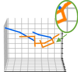
H36M
