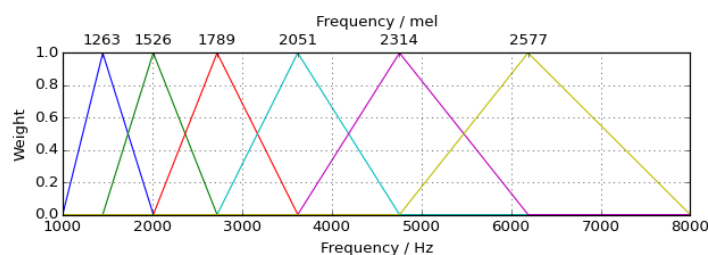
Figura 4.4: Filtre Mel
