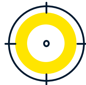
o3
