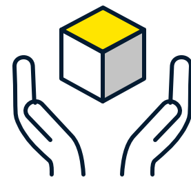
GPT-4o (o4)
