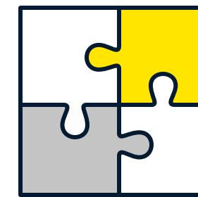
GPT-3.5
