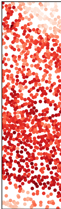
TAVIE-SSG
