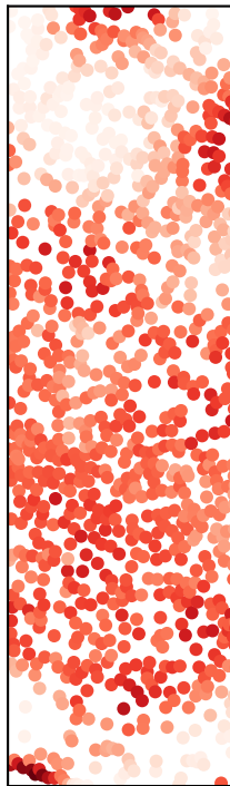
ADVI (FR)
