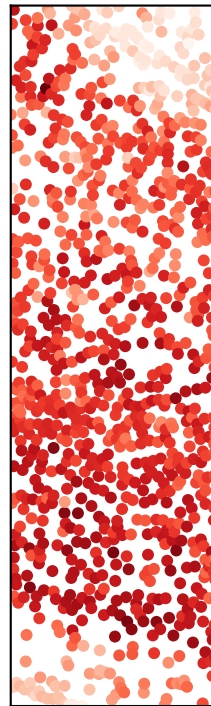
PyMC (NUTS)
