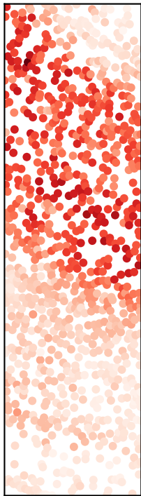
TAVIE-SSG
