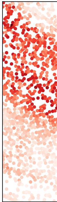
PyMC (NUTS)
