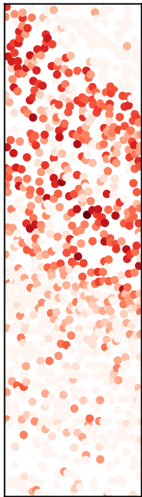
True
