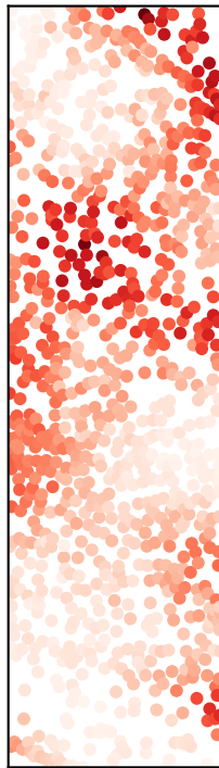
ADVI (FR)
