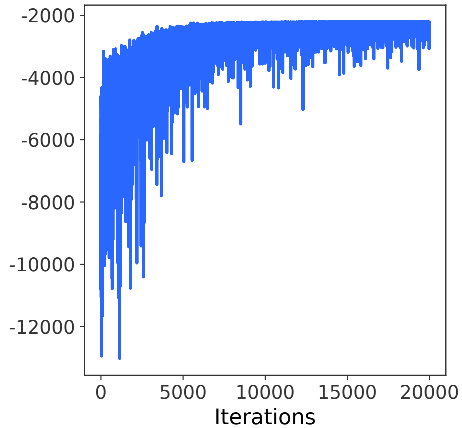
ADVI (FR)
