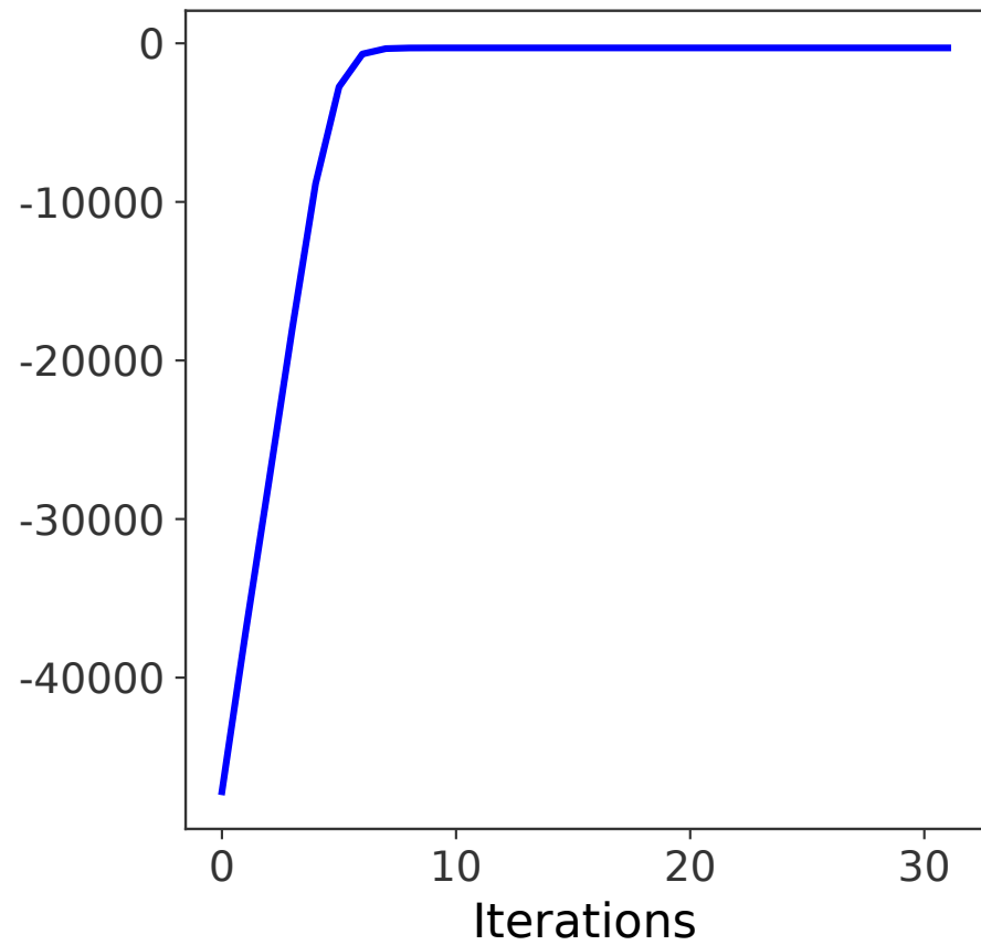
TAVIE-SSG
