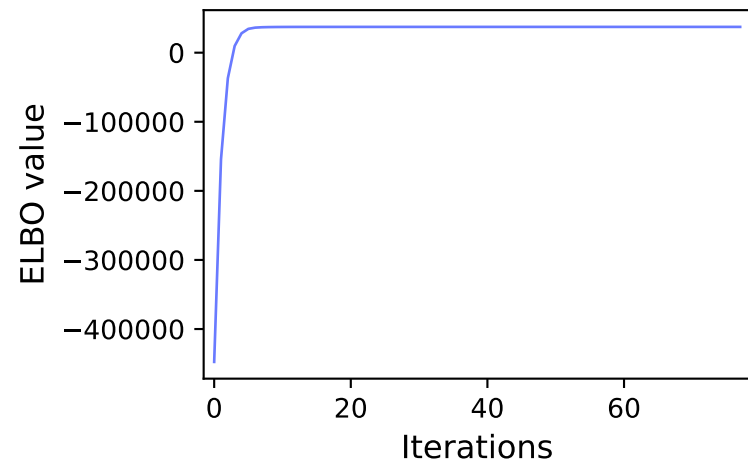
Quantile = 0.70
