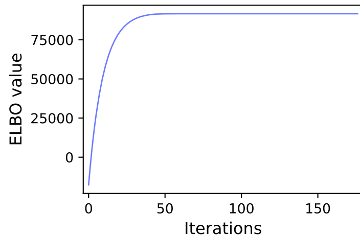
Quantile = 0.95
