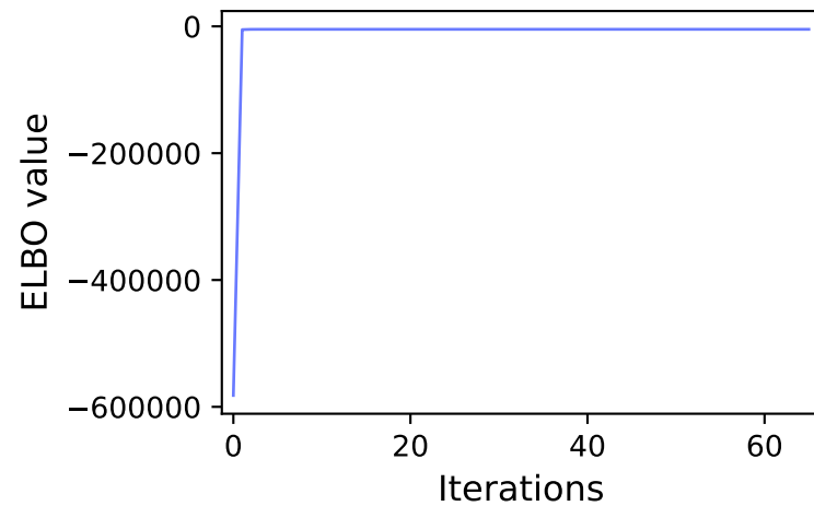
Quantile = 0.95
