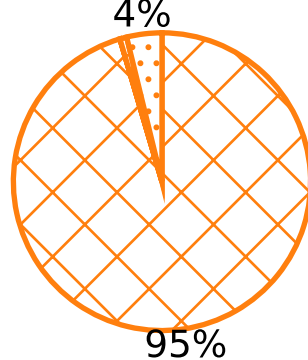
SIFT
