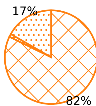
Text2Image
