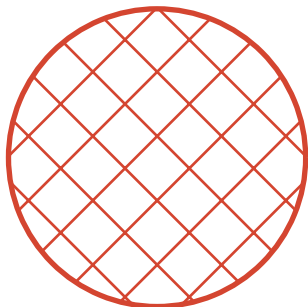
SpaceV
