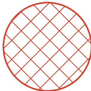
Text2Image
