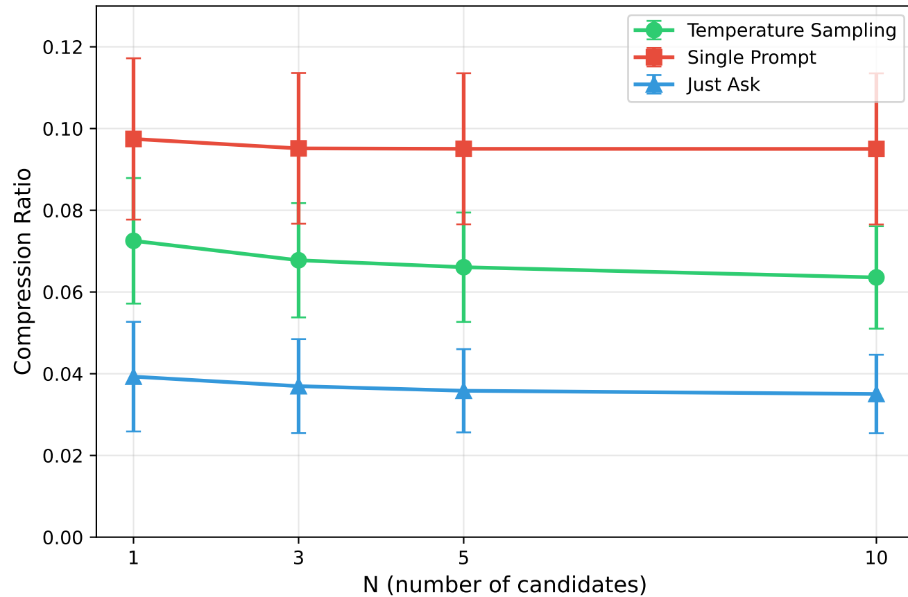
AIME
