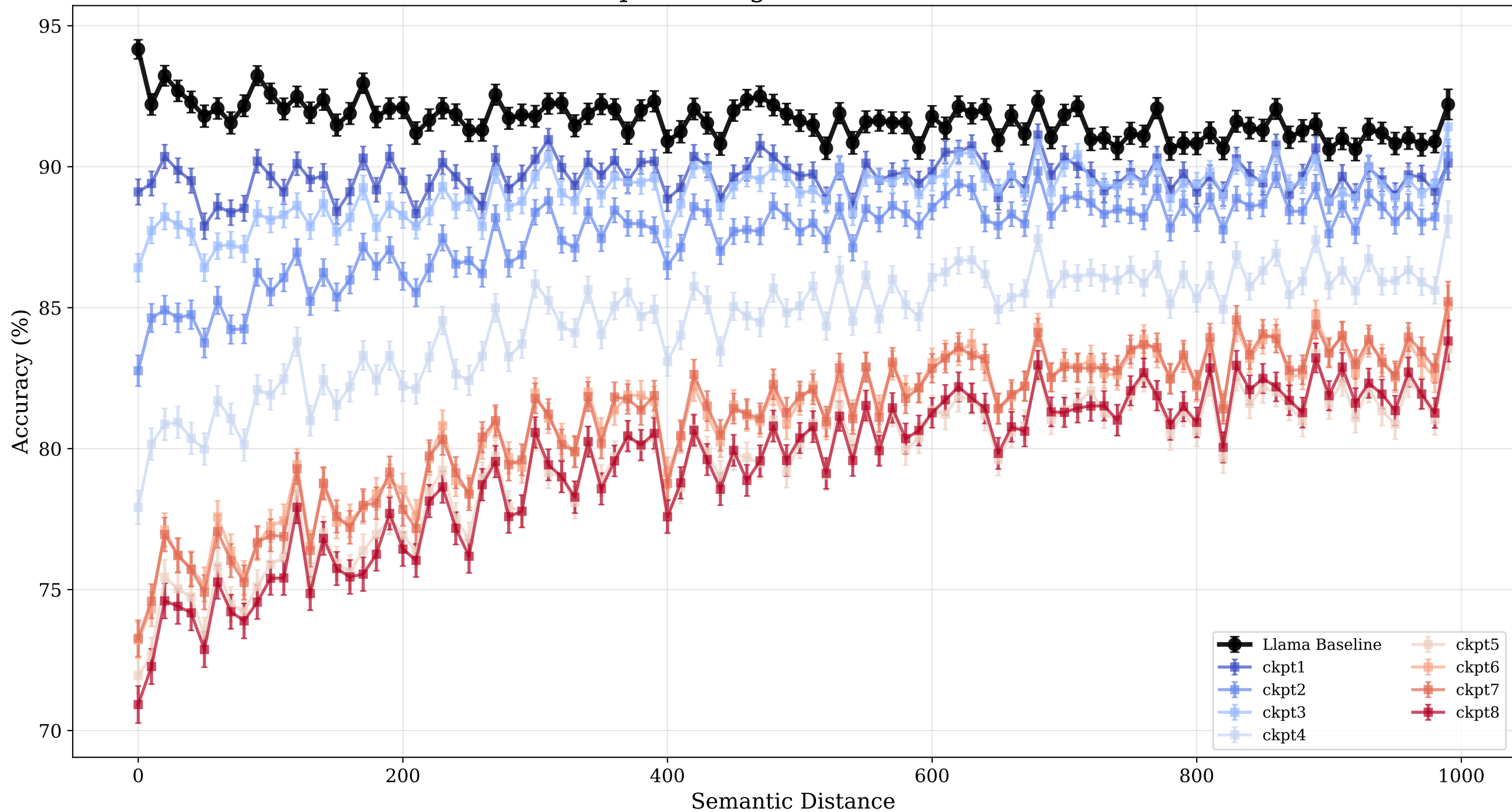
Checkpoint Progression: Llama-RMU
