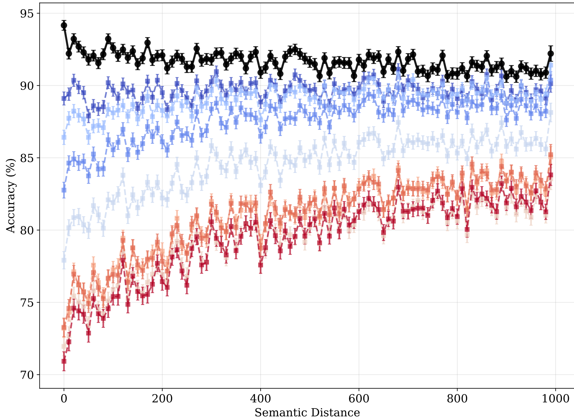
RMU
