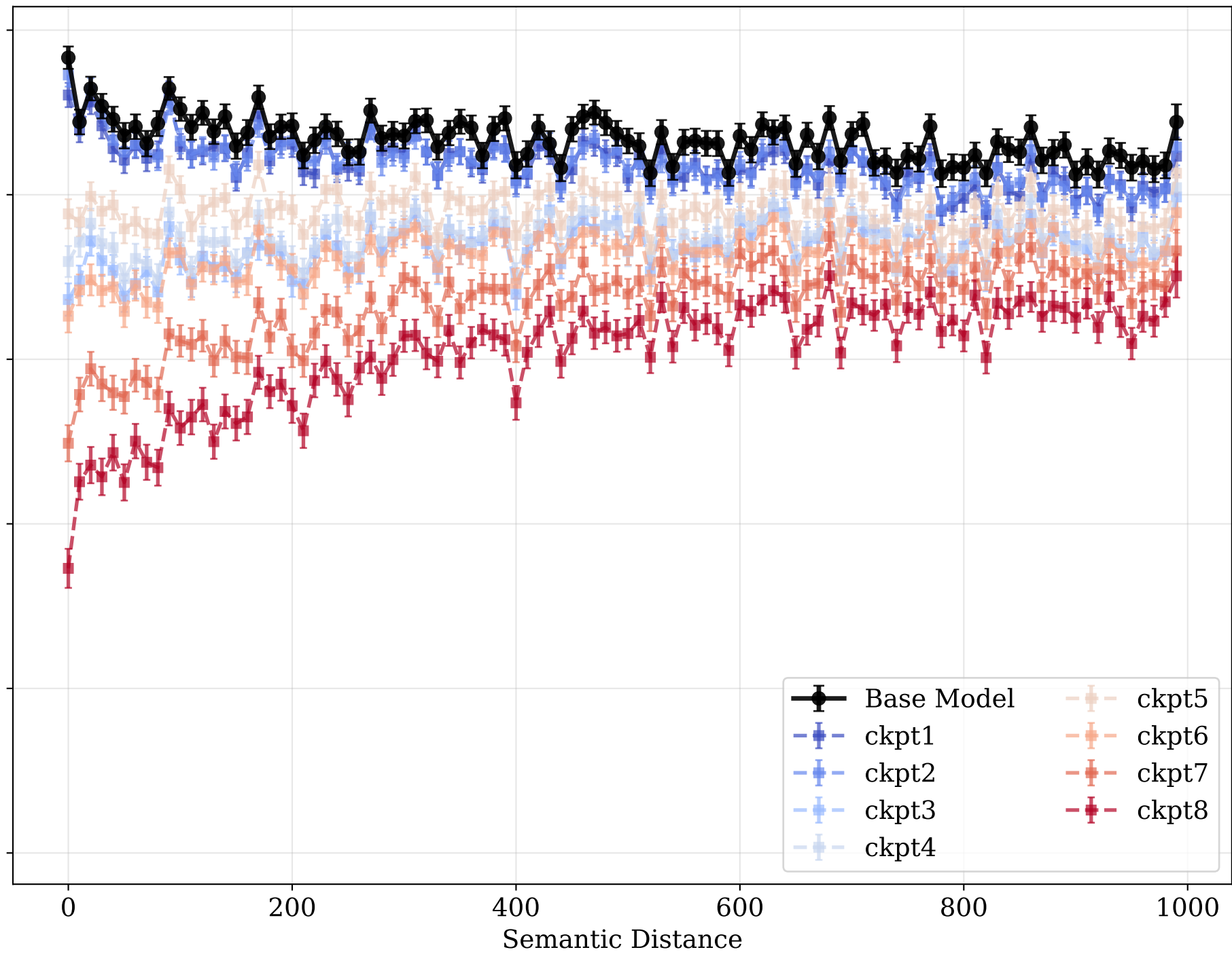
ELM
