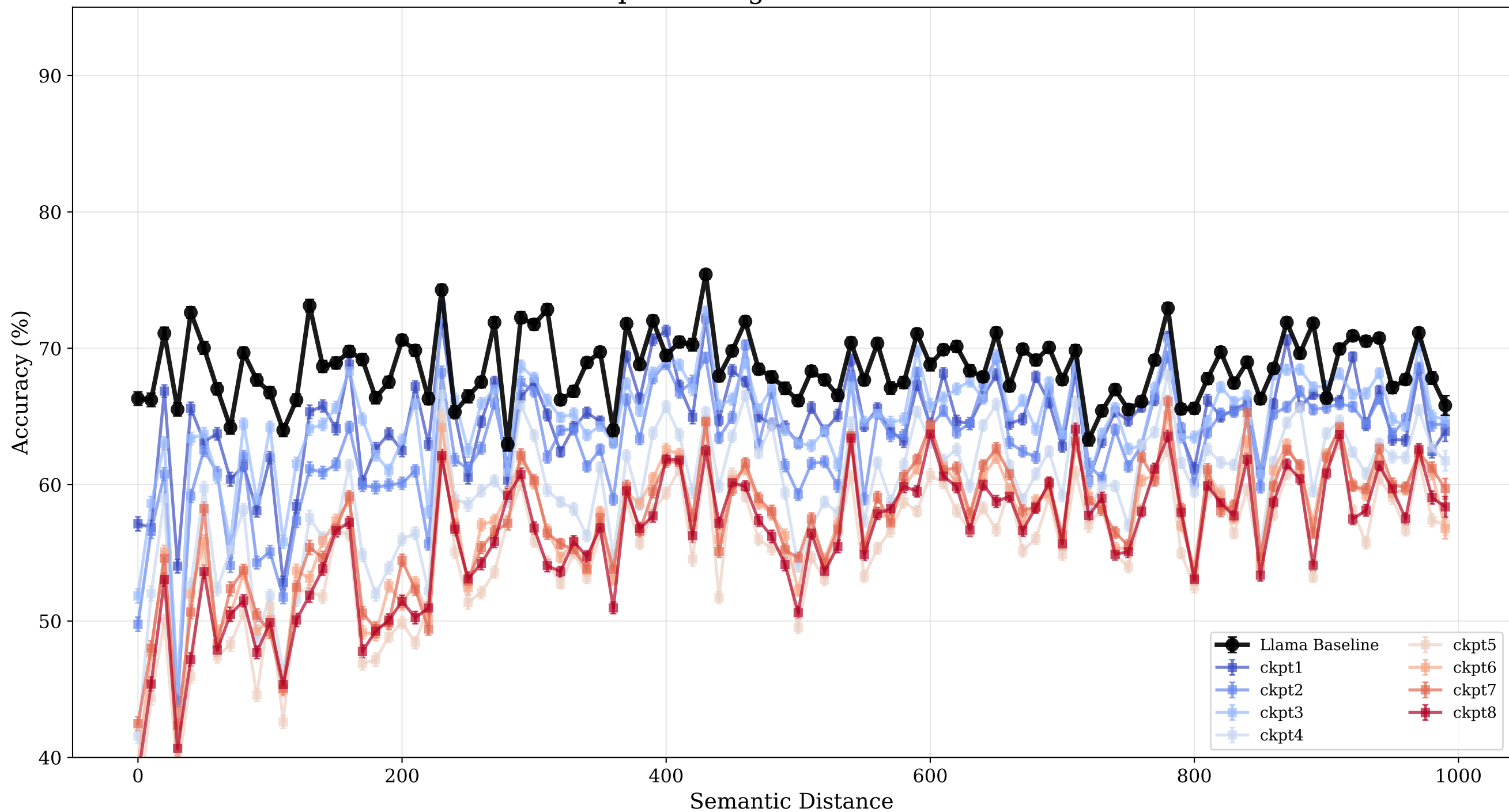
Checkpoint Progression: Llama-RMU
