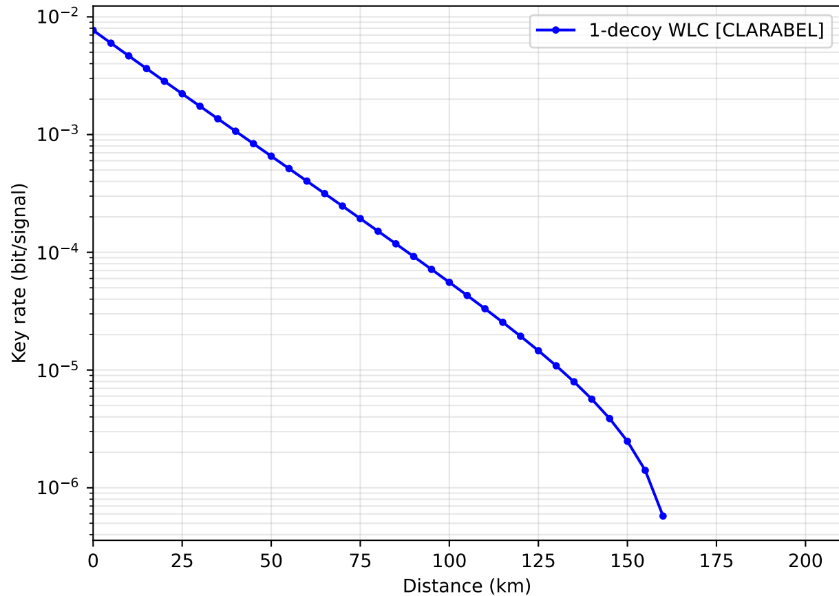
Decoy-state BB84 — Lo-Ma-Chen 2005 parameters
