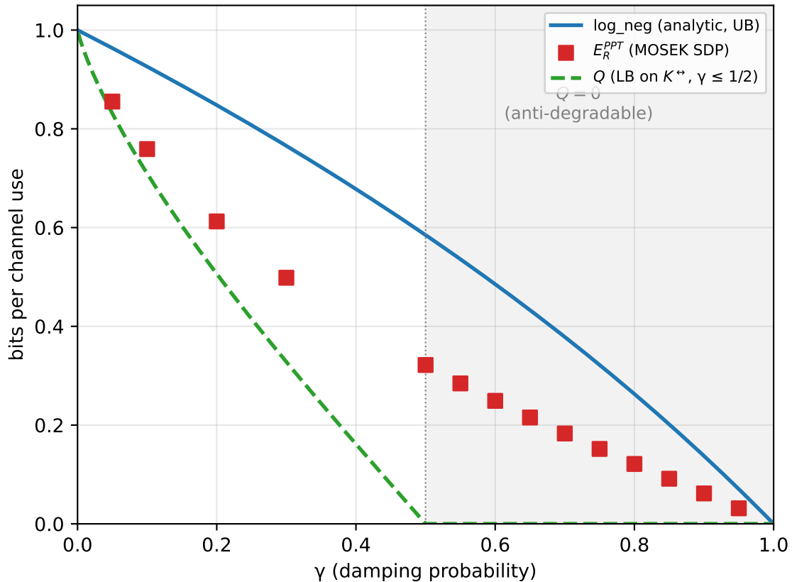
AD hierarchy: Q \leq K^{\leftrightarrow} \leq E_R^{PPT} \leq \log \|\cdot\|_{PT}
