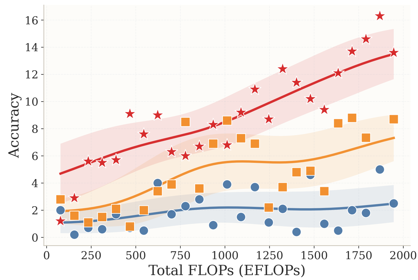
OBQA
