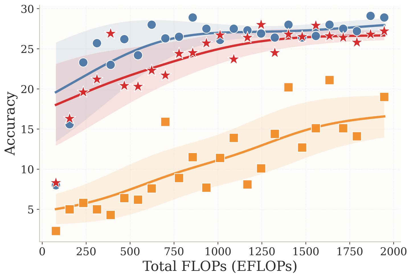
SIQA
