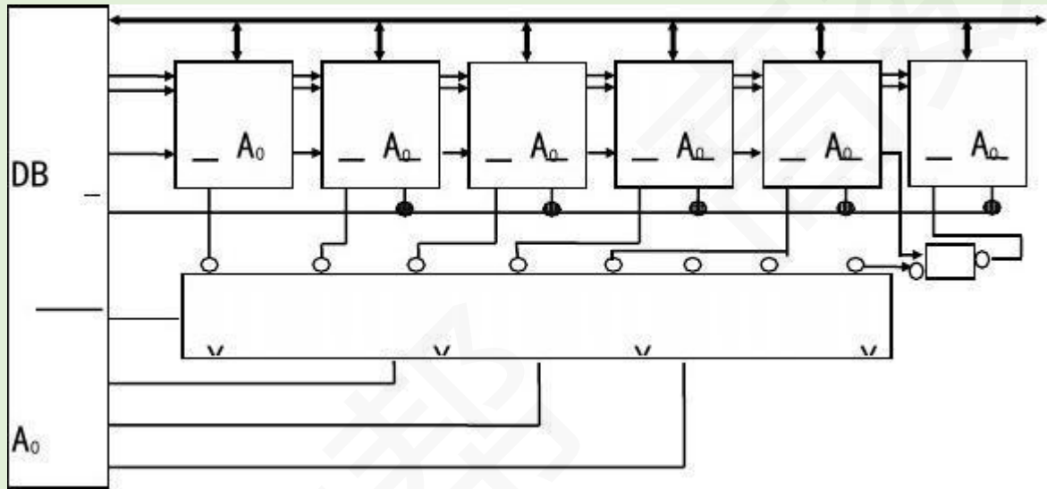
图 2 主存地址分布及芯片连接图
