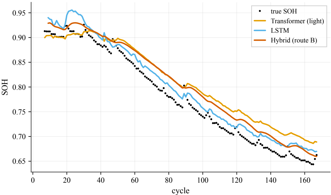
SOH trajectory (held-out B0005)
