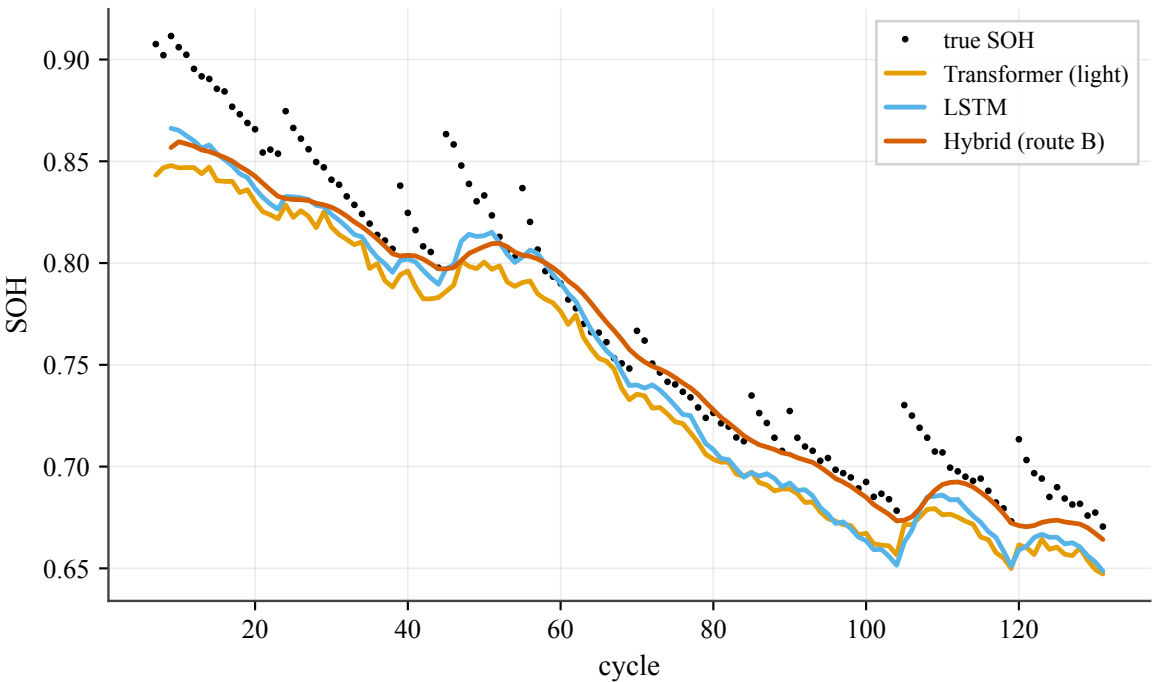
SOH trajectory (held-out B0018)
