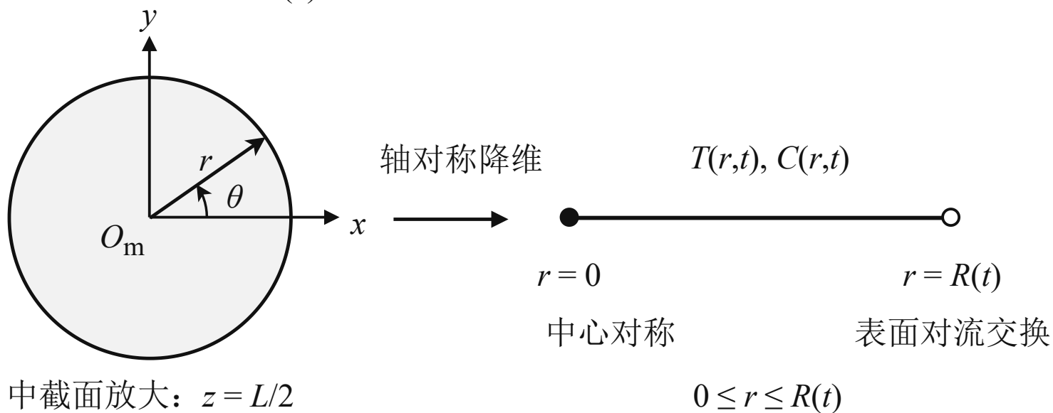
(a) 初始圆柱几何与坐标系
