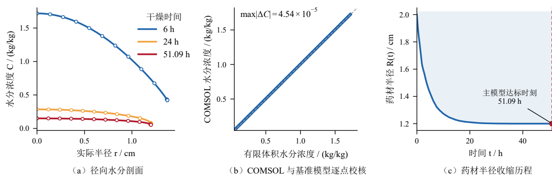
图 13 加密 COMSOL 有限元与有限体积解的剖面对照及半径收缩历程
