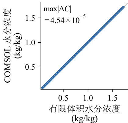
(b) COMSOL 与基准模型 逐点校核
