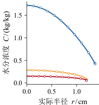
(a) 径向水分剖面
