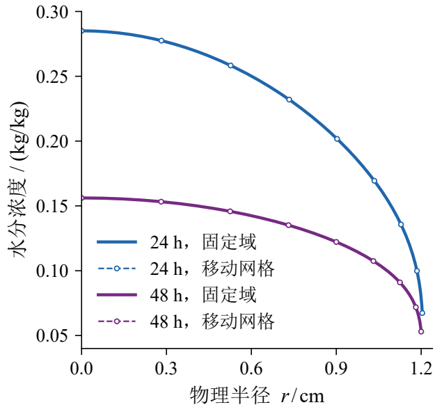
(b) 完整径向剖面
