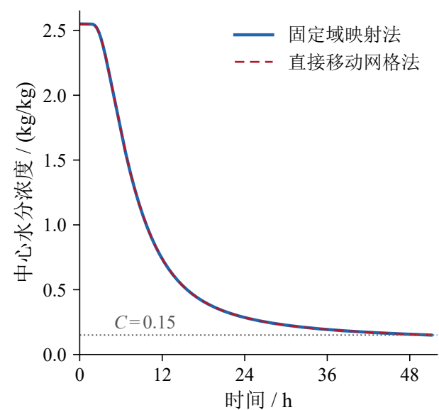
(a) 中心水分轨迹
