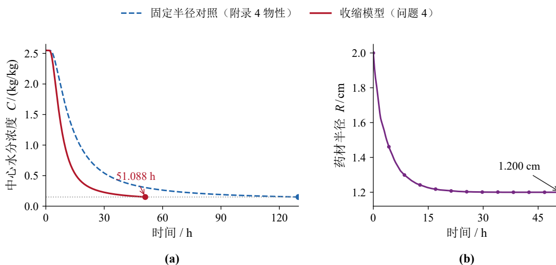
图 11 问题四收缩与固定半径反事实比较
