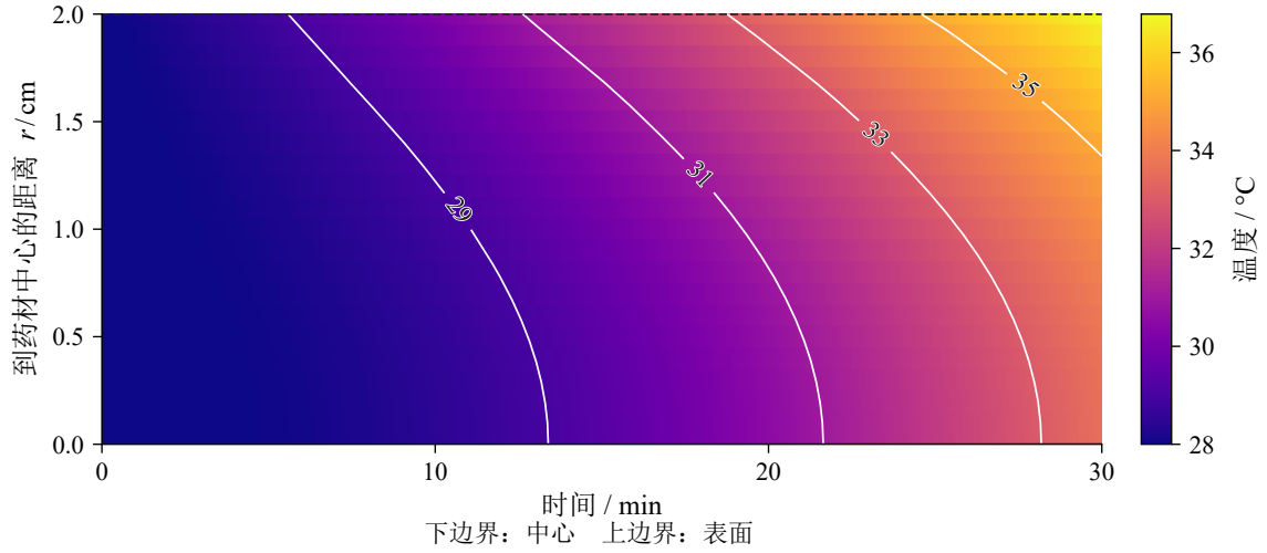
图 4 问题一预热温度的时空分布及等温线 (0–30 min)
