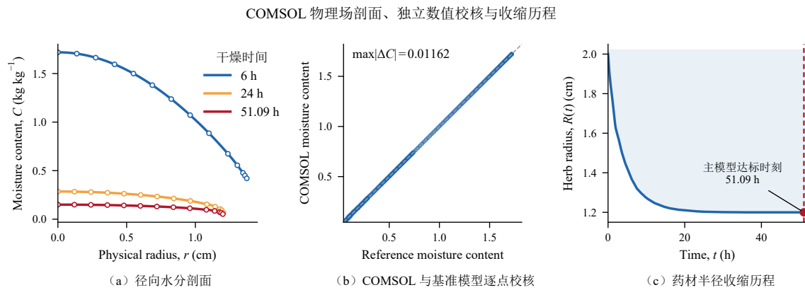
图 13 COMSOL 有限元剖面、原有限体积结果校核与半径收缩历程
