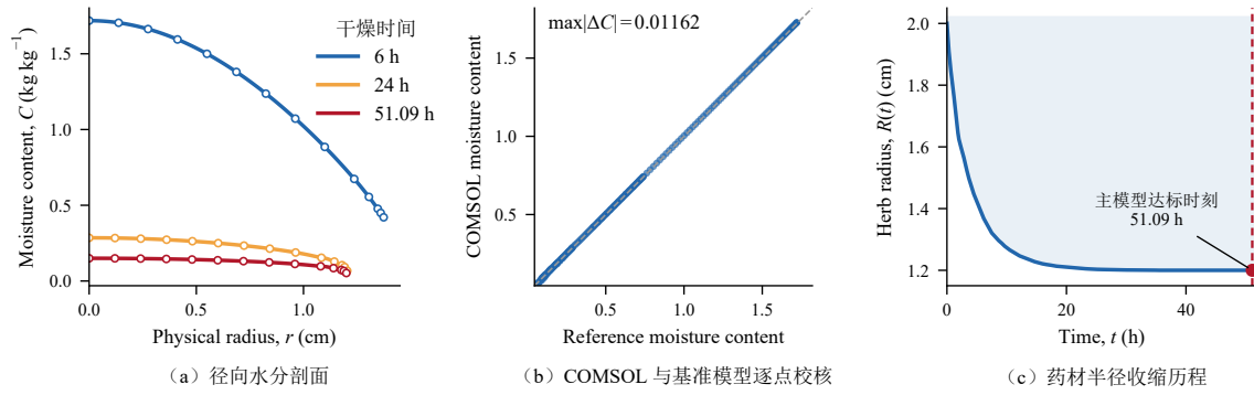
图 13 COMSOL 有限元剖面、原有限体积结果校核与半径收缩历程
